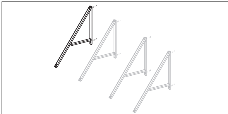
Abb. 5.5 Gestelle ausrichten
