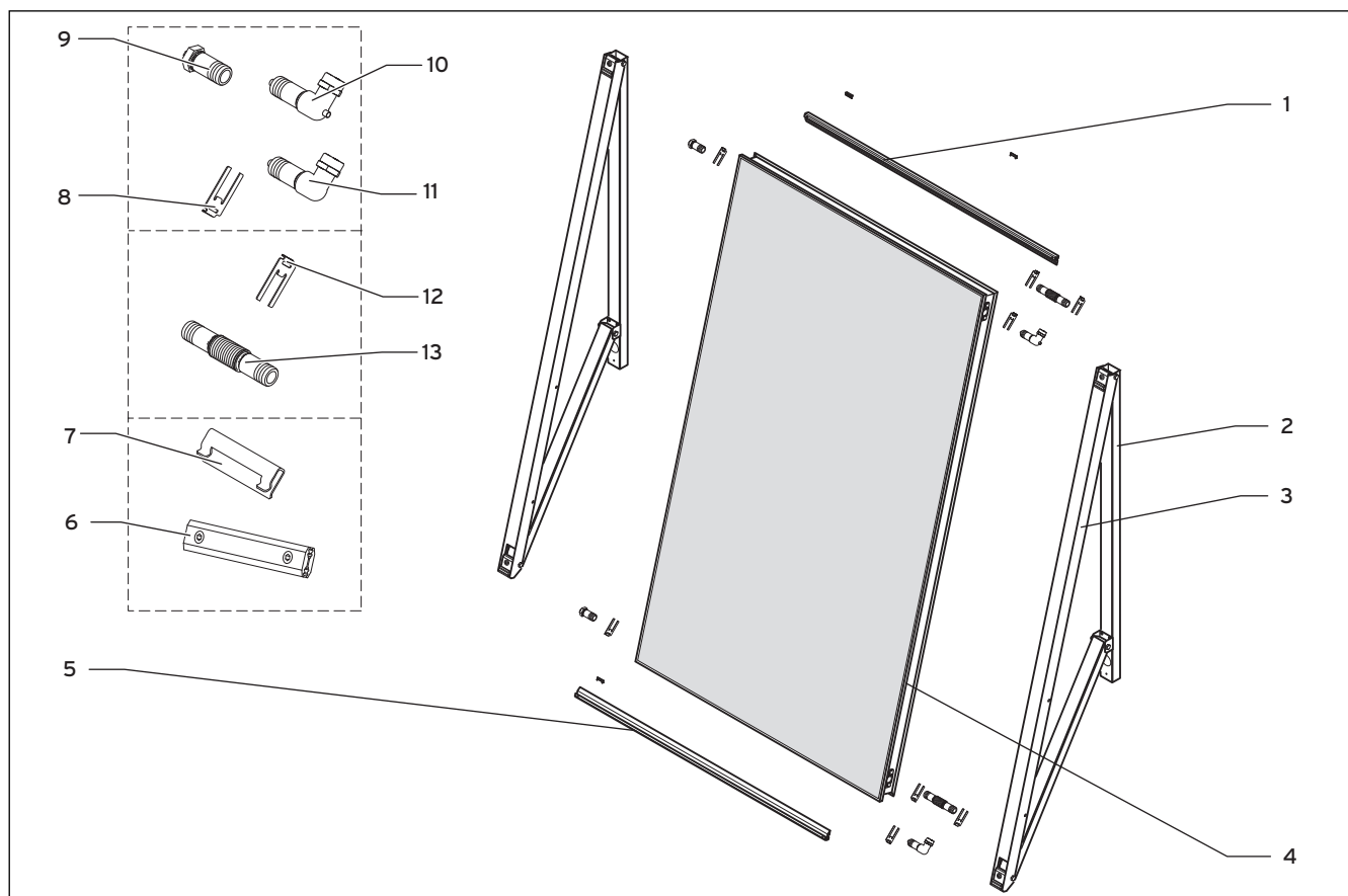
Abb. 5.2 Einbauset
