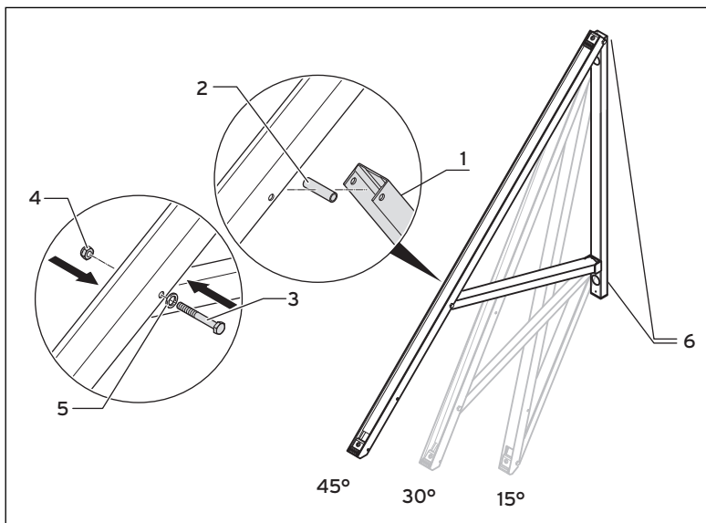
Abb. 5.4 Gestell montieren
