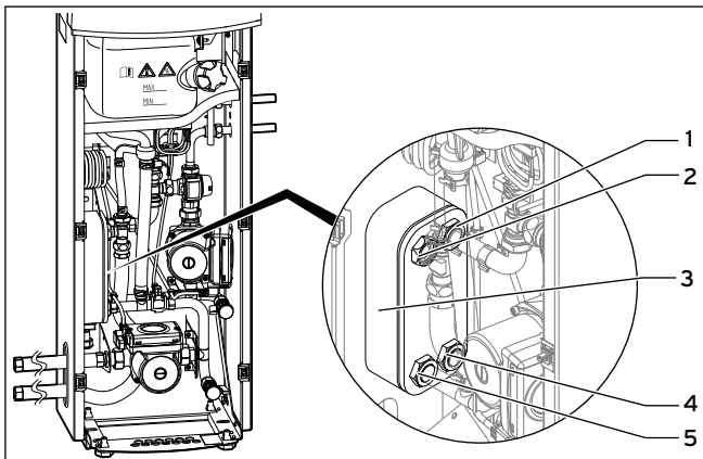
10.5 Wärmetauscher
