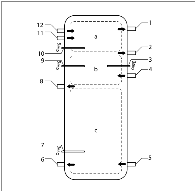
5.7 Prinzipdarstellung beliebiger Pufferspeicher (System ecoPOWER 1.0 HS 2)
