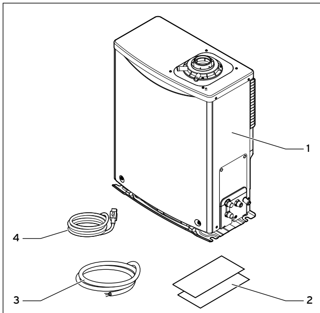
4.2 Lieferumfang Verpackungseinheit 1: KWK-Modul
