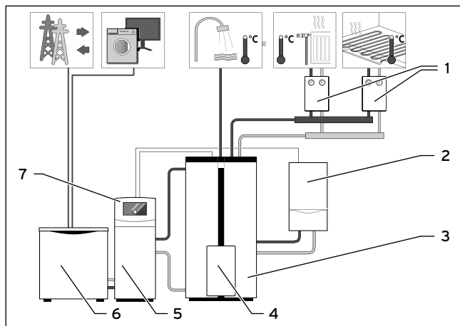
3.1 Prinzipdarstellung System ecoPOWER1.0 HS1
