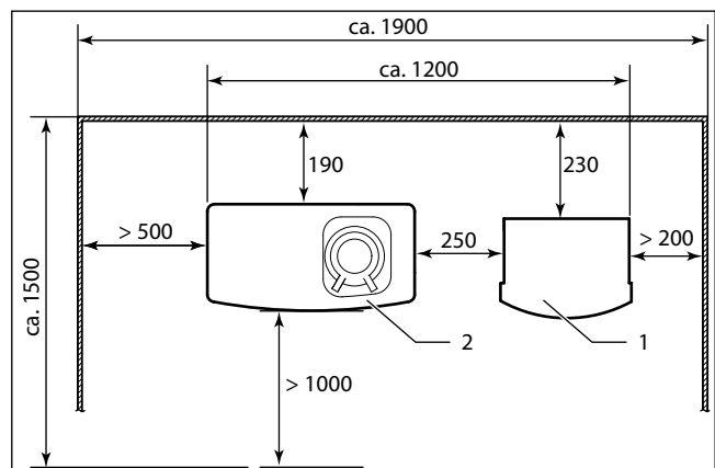
4.1 Abstände, Mindestabstände und Wartungsfreiräume für das mikro-BHKW
