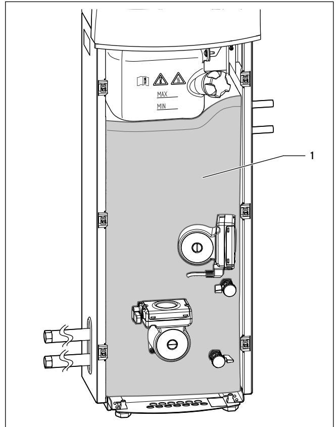
7.1 Wärmeauskopplungsmodul mit Front-Isoliermatte
