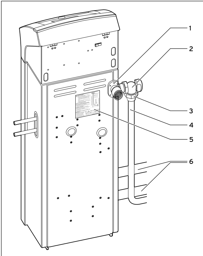
4.11 Rückansicht Wärmeauskopplungsmodul/Systemregler
