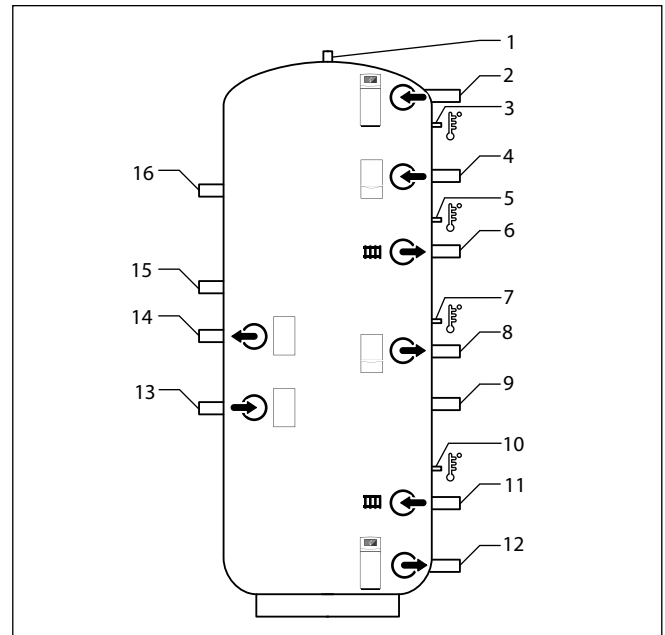
5.6 Prinzipdarstellung Pufferspeicher allSTOR (System ecoPOWER 1.0 HS1)
