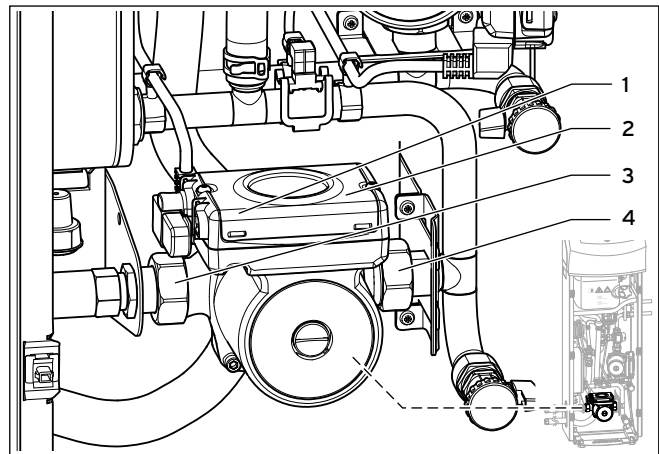
10.4 Kühlmittelpumpe
