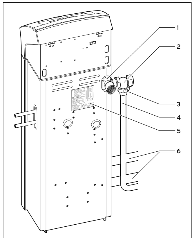
4.13 Rückansicht Wärmeauskopplungsmodul/Systemregler
