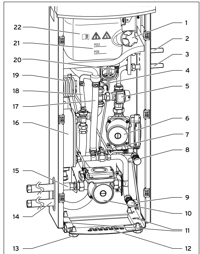
5.8 Wärmeauskopplungsmodul
