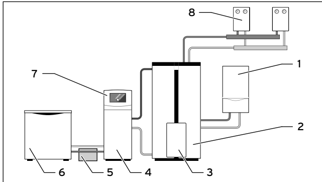
4.7 Anordnung der Systemkomponenten System ecoPOWER1.0 HS 1
