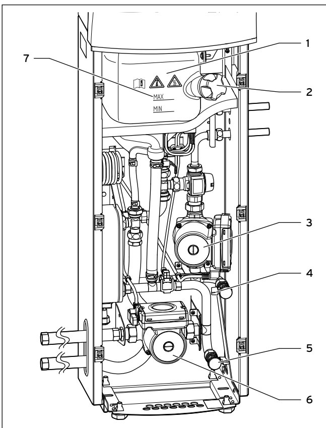
7.2 Kühlmittelbehälter befüllen
