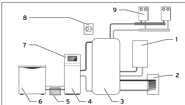
4.8 Anordnung der Systemkomponenten System ecoPOWER1.0 HS 2
