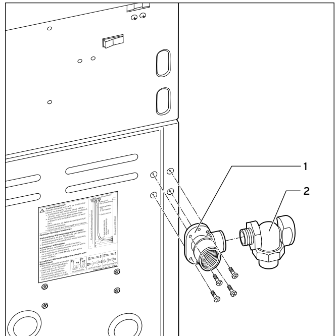
4.12 Wandscheibe und Gasabsperrhahn an das Wärmeauskopplungsmodul montieren
