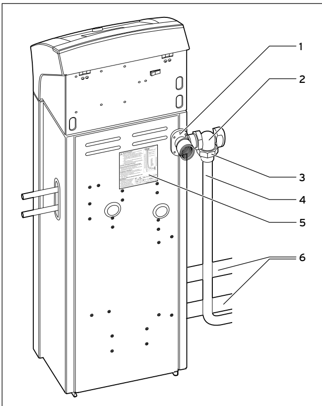
10.8 Rückansicht Wärmeauskopplungsmodul/Systemregler
