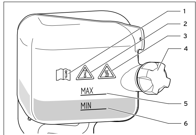
9.1 Kühlmittelbehälter
