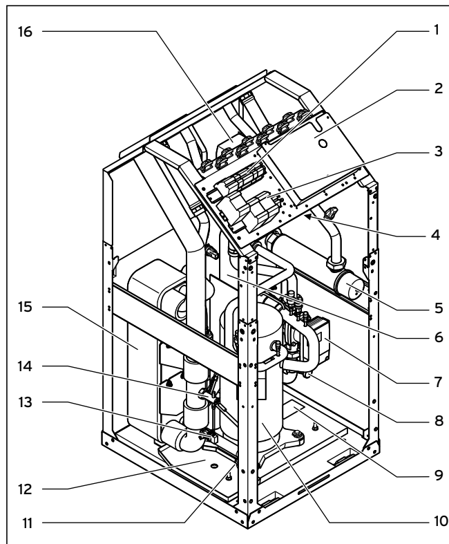
3.6 Vorderansicht geöffnet (VWW)
