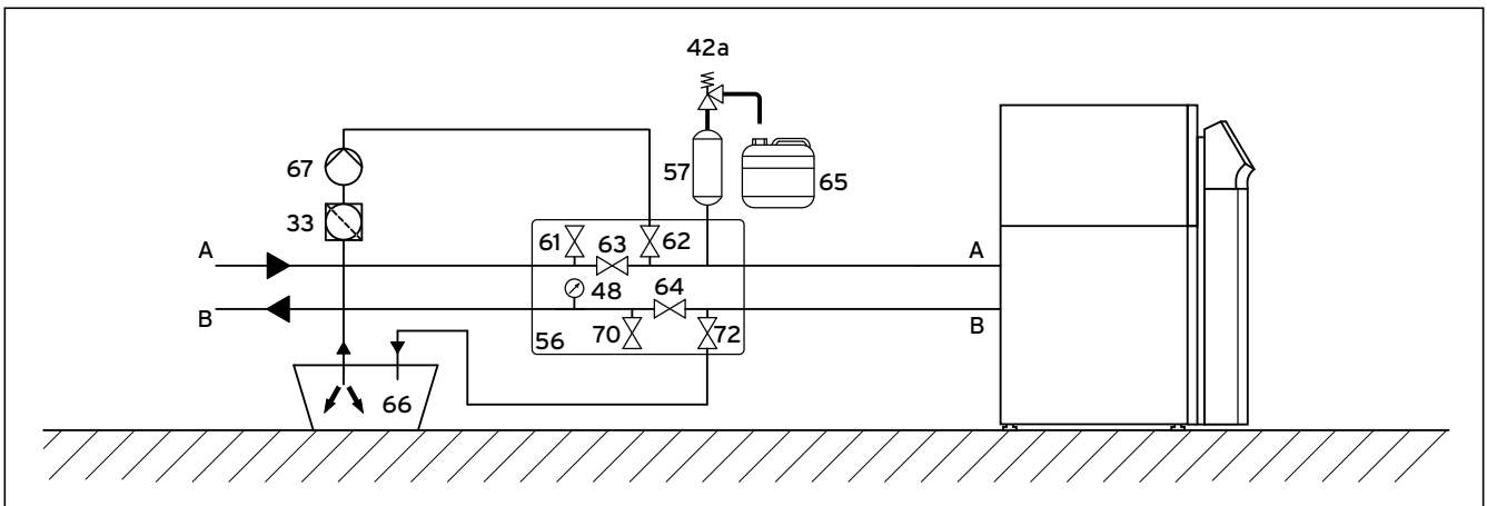
6.5 Inneren Teil des Solekreises befüllen und entlüften
