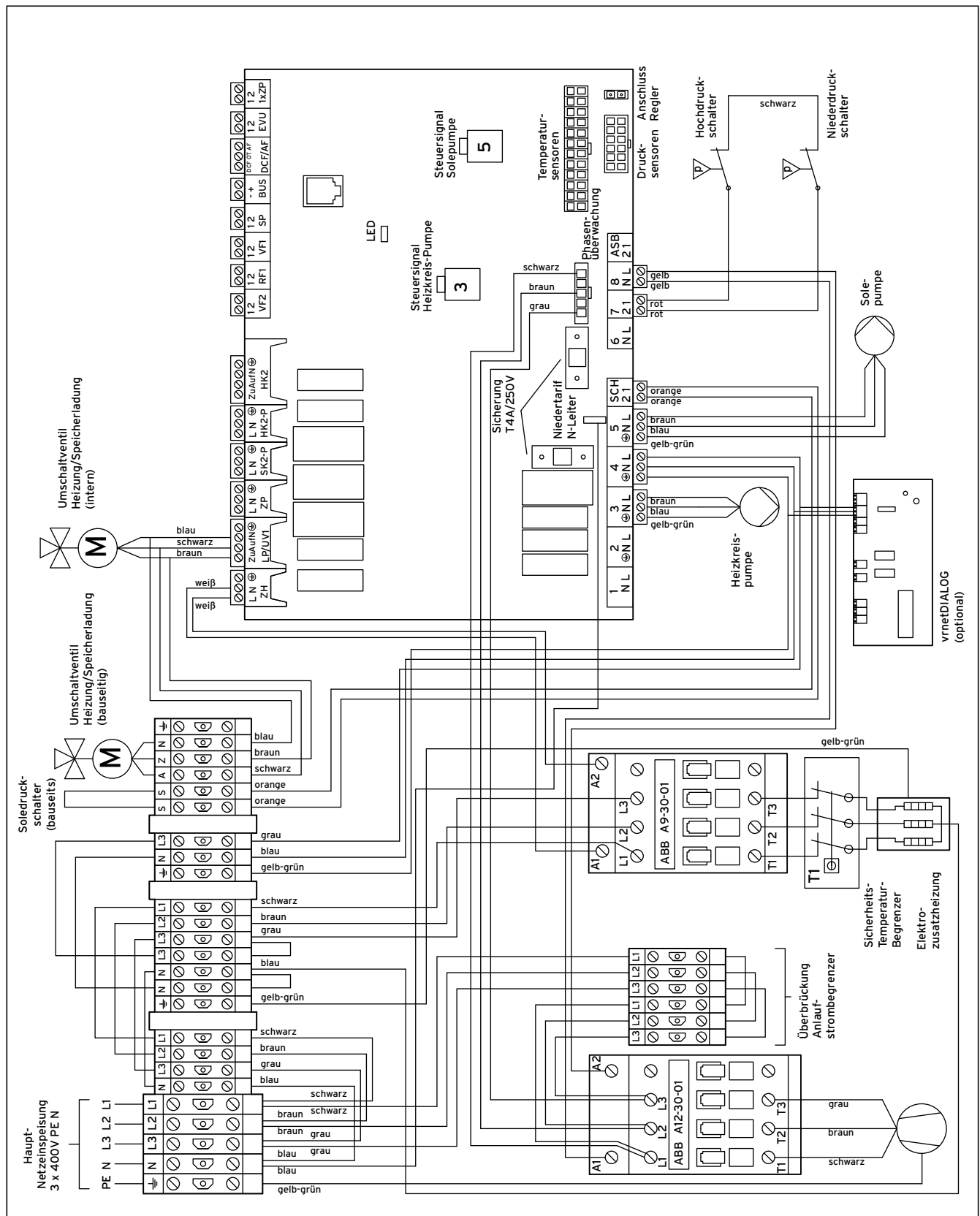
17.3 Stromlaufplan VWS 61/3 - VWS 141/3
