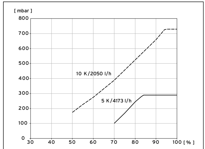
9.15 Diagramm Leistungsoptimierung Heizkreispumpe VWW 171/3
