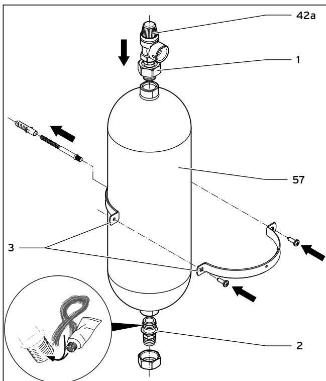
5.8 Sole-Ausgleichsbehälter montieren
