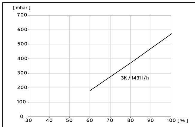
9.1 Diagramm Leistungsoptimierung Solepumpe VWS 61/3
