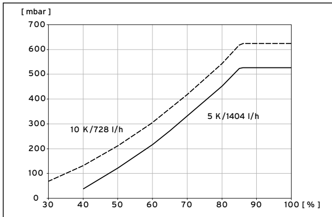
9.11 Diagramm Leistungsoptimierung Heizkreispumpe VWW 61/3
