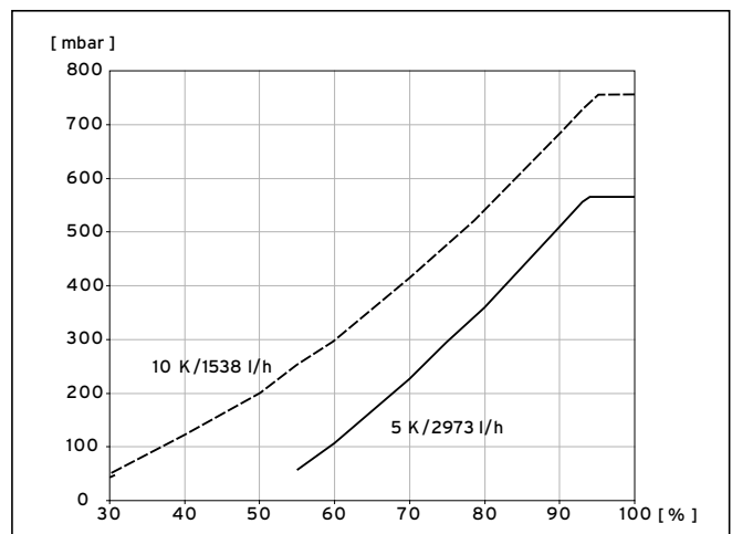
9.10 Diagramm Leistungsoptimierung Heizkreispumpe VWS 171/3
