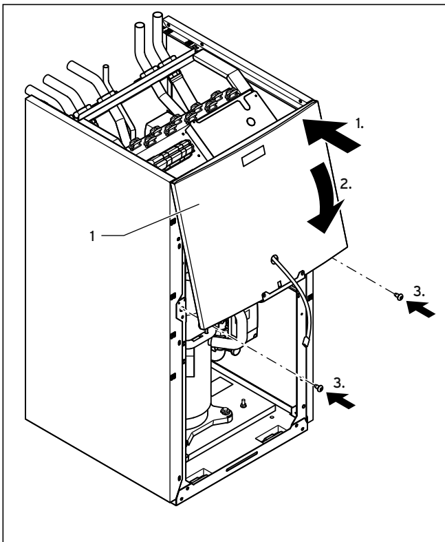
7.18 Oberteil der Frontverkleidung montieren
