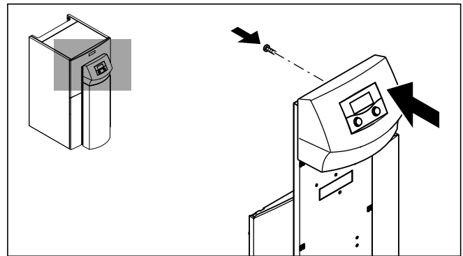
7.19 Bedienkonsole montieren
