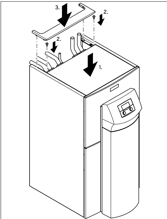
7.23 Obere Verkleidungsteile montieren
