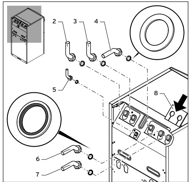
5.6 Anschlusswinkel montieren
