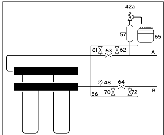
5.7 Armaturen im Solekreis
