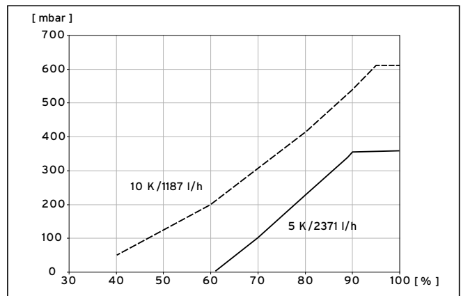
9.9 Diagramm Leistungsoptimierung Heizkreispumpe VWS 141/3
