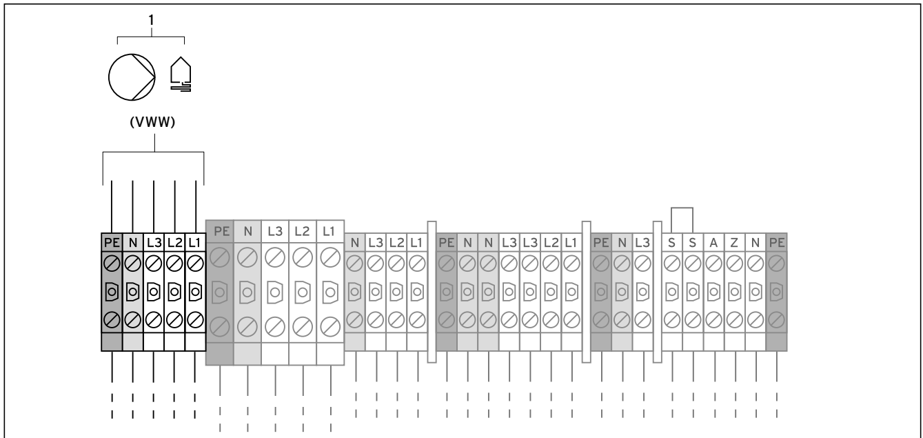
7.7 Externen Brunnenpumpe anschließen (nur VWW)
