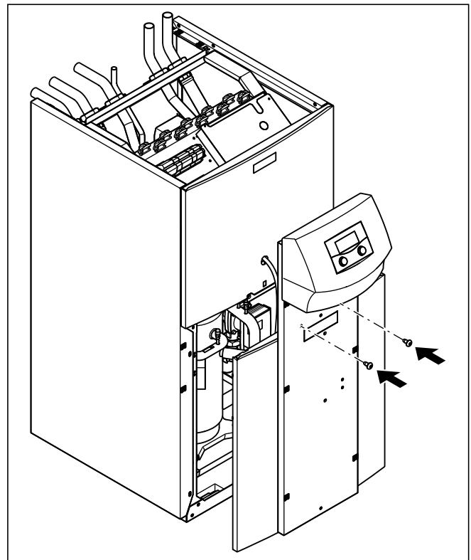
7.20 Unterteil der Frontverkleidung montieren
