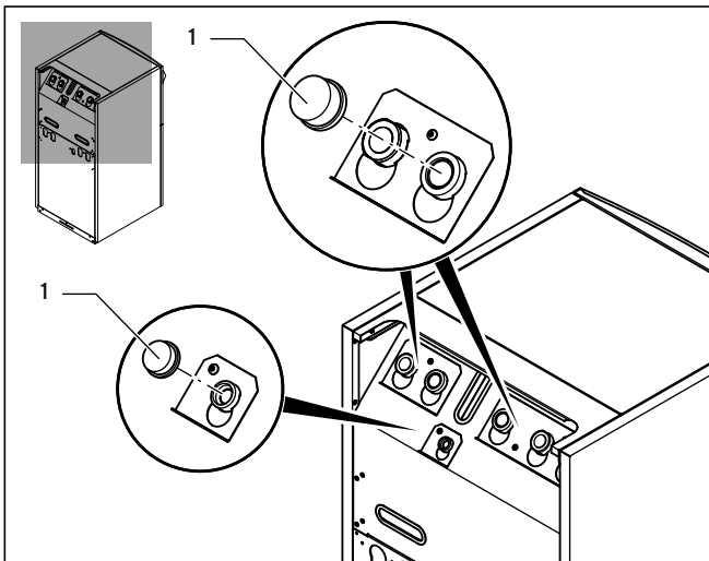
5.5 Blindkappen entfernen
