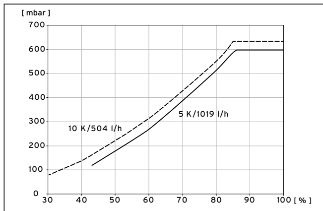
9.6 Diagramm Leistungsoptimierung Heizkreispumpe VWS 61/3
