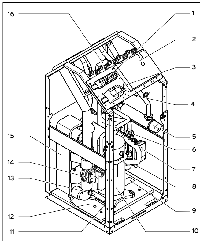
3.5 Vorderansicht geöffnet (VWS)
