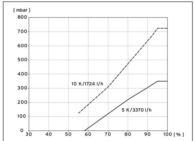
9.14 Diagramm Leistungsoptimierung Heizkreispumpe VWW 141/3
