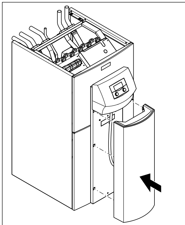
7.22 Abdecksäule der Bedienkonsole montieren
