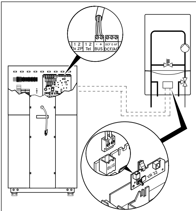
7.16 Heizgerät mit eBUS-Schnittstelle anschließen
