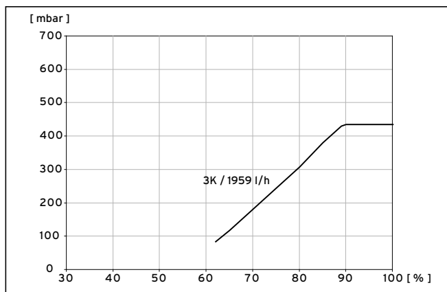
9.2 Diagramm Leistungsoptimierung Solepumpe VWS 81/3
