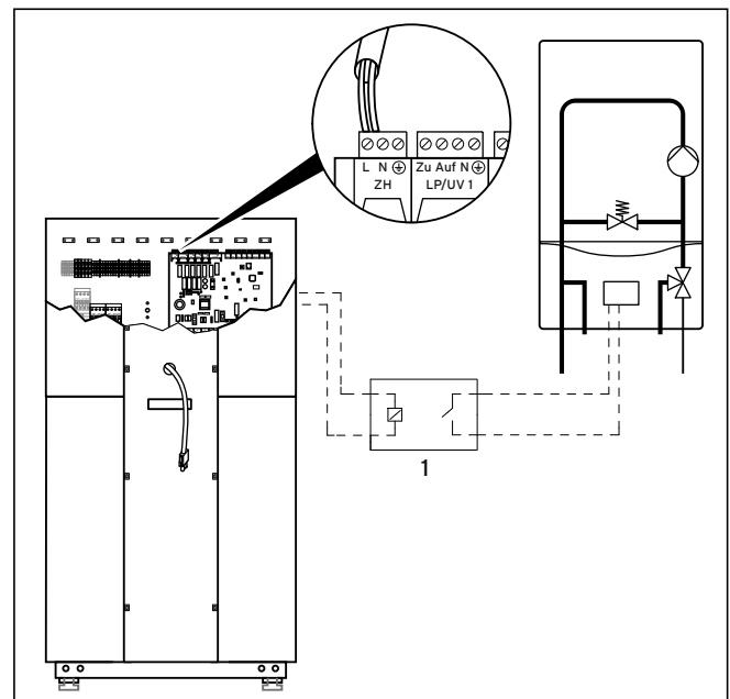
7.17 Heizgerät ohne eBUS-Schnittstelle anschließen
