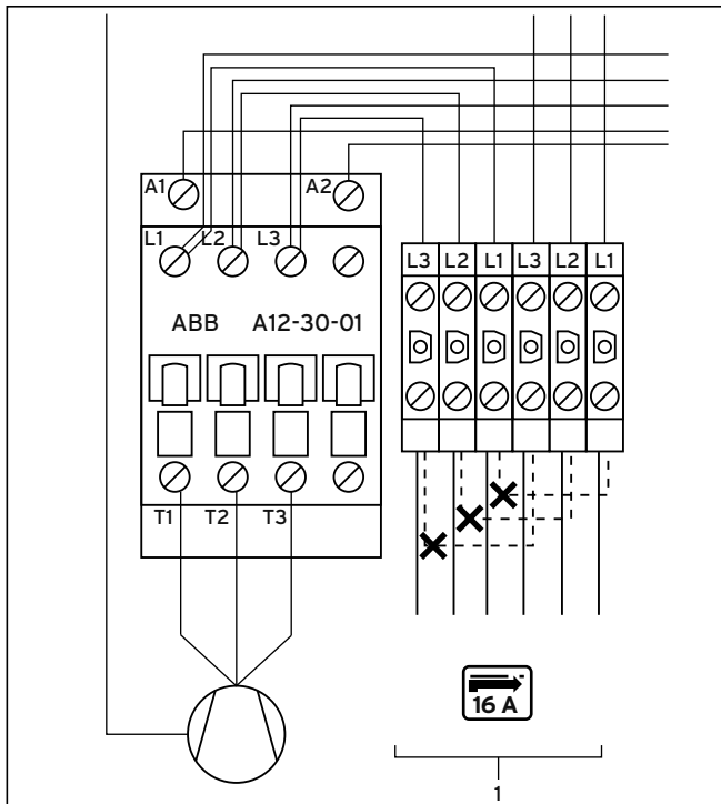
7.10 Anlaufstrombegrenzer (Zubehör) anschließen
