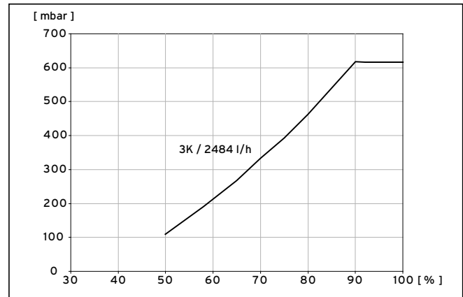
9.3 Diagramm Leistungsoptimierung Solepumpe VWS 101/3
