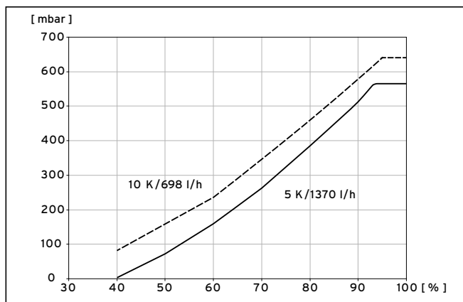
9.7 Diagramm Leistungsoptimierung Heizkreispumpe VWS 81/3
