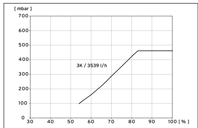
9.4 Diagramm Leistungsoptimierung Solepumpe VWS 141/3
