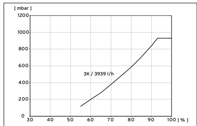
9.5 Diagramm Leistungsoptimierung Solepumpe VWS 171/3
