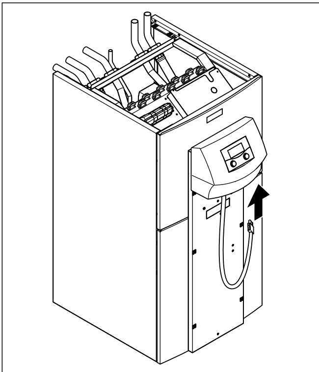
7.21 eBUS-Leitung der Bedienkonsole anschließen
