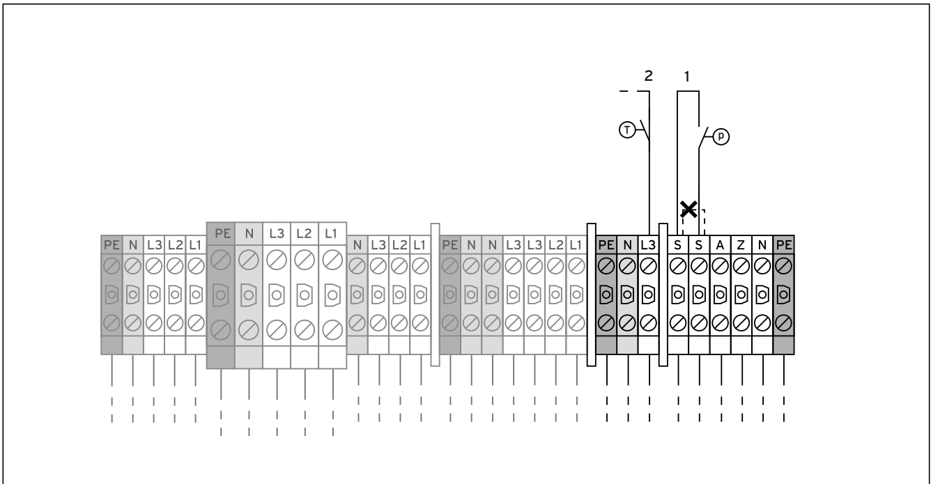
7.8 Externen Soledruckschalter (nur VWS) und Maximalthermostaten anschließen
