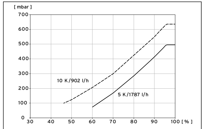
9.8 Diagramm Leistungsoptimierung Heizkreispumpe VWS 101/3
