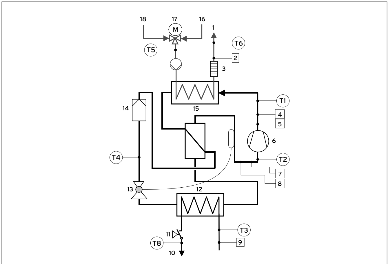
17.2 Wärmepumpenschema VWW ..1/3
