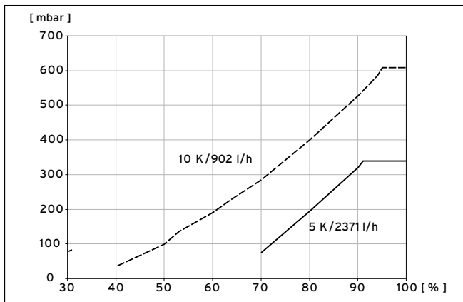
9.13 Diagramm Leistungsoptimierung Heizkreispumpe VWW 101/3
