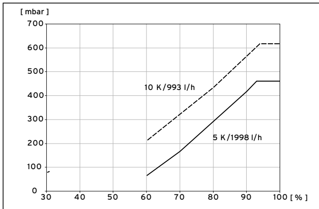
9.12 Diagramm Leistungsoptimierung Heizkreispumpe VWW 81/3
