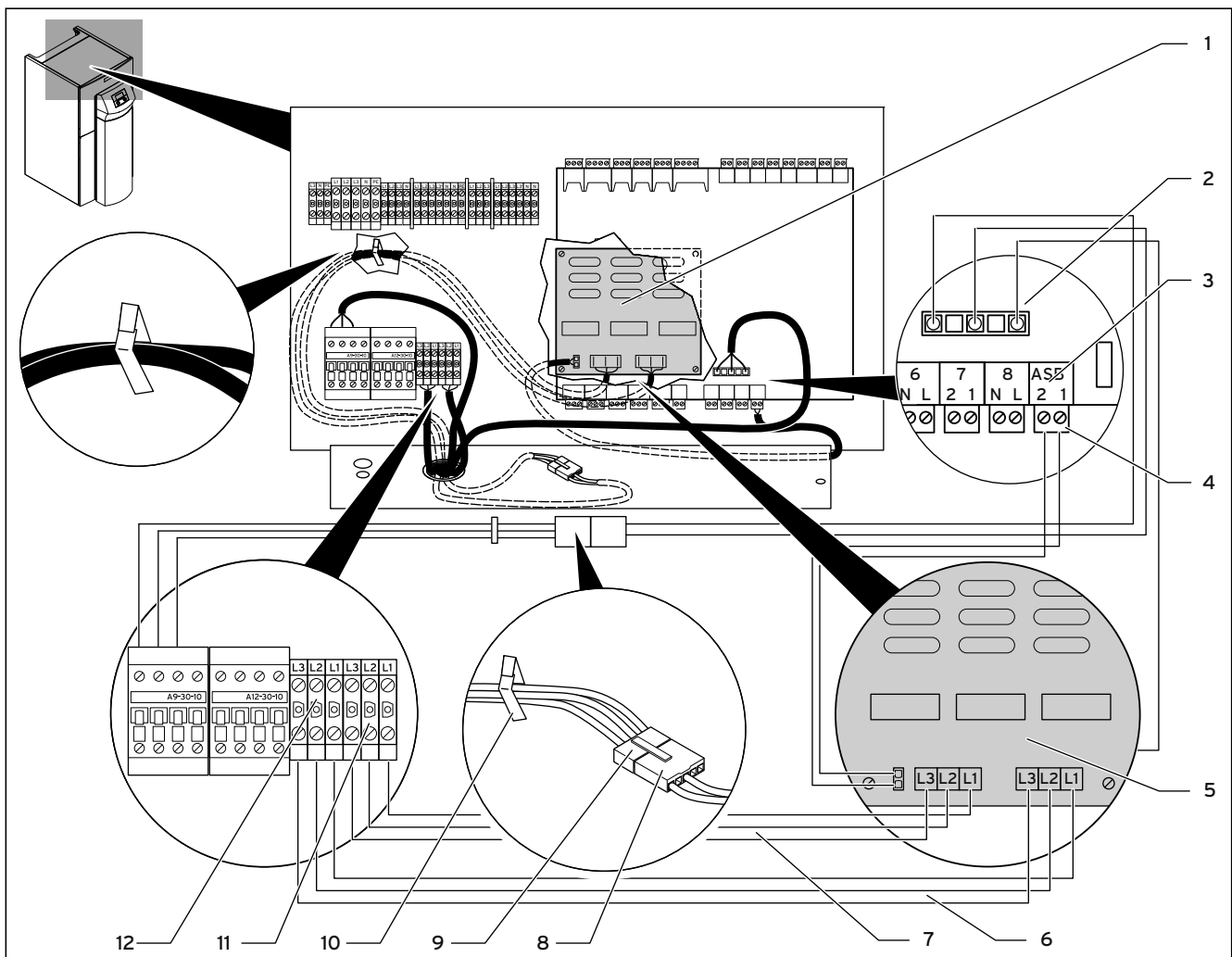
Fig. 4.6 Raccordement à geoTHERM VWS/VWW/VWL-S ..1 et VWS ..4
