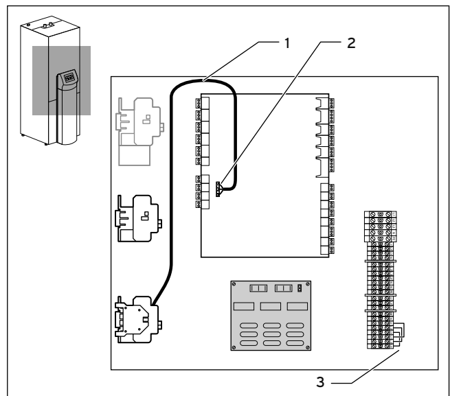
Fig. 4.8 Démontage de la surveillance des phases du compresseur VWS/VWW/VWL-S ..2 und VWS ..3
