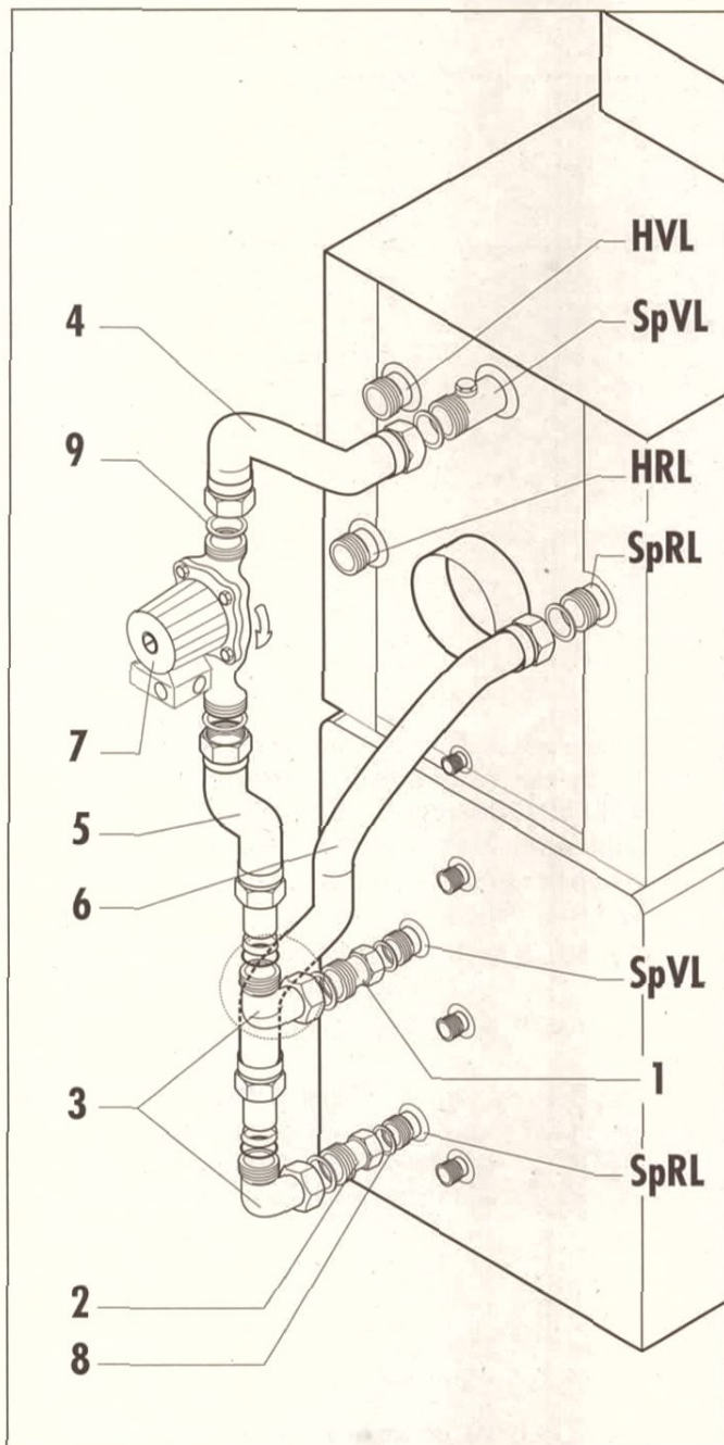
Abb. 1 Montage Speicherladeset Art.-Nr. 305 837
