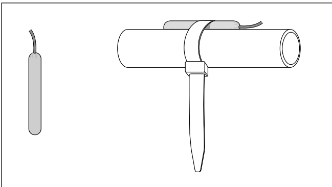
4.9 Standardfühler VR 10 als Anlegefühler
