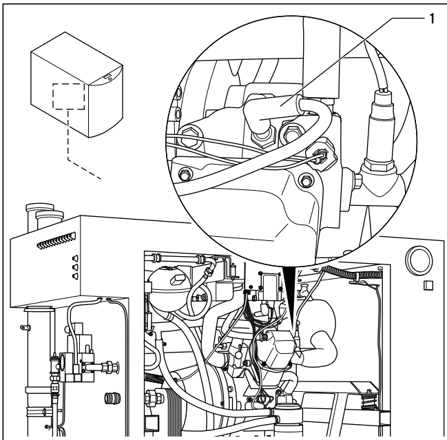
9.1 Zündkabel und Zündkerze auswechseln
