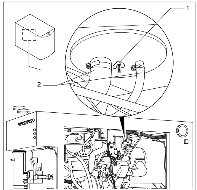
9.2 Luftfilter auswechseln
