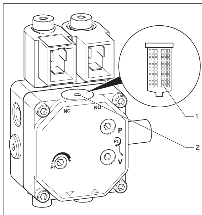
1 Ölpumpenfilter 2 Verschlusschraube
