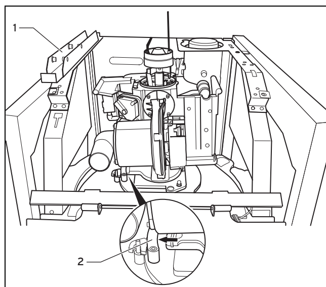
1 Ablageposition 2 Verriegelungsnase
