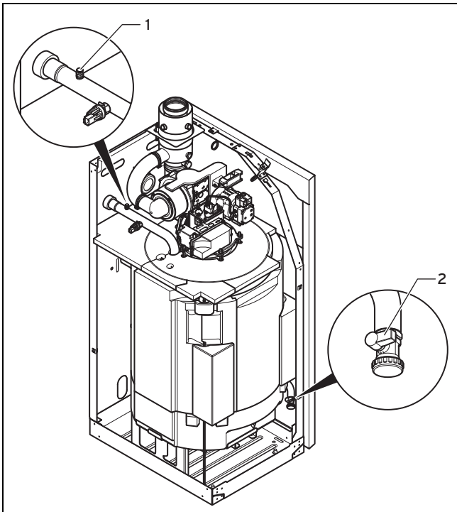
1 Entlüftungsnippel
