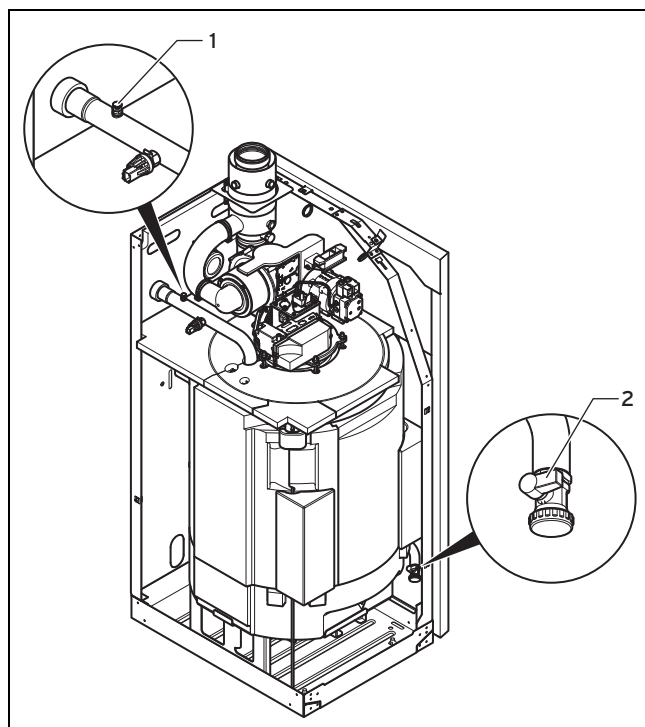
1 Entlüftungsnippel
