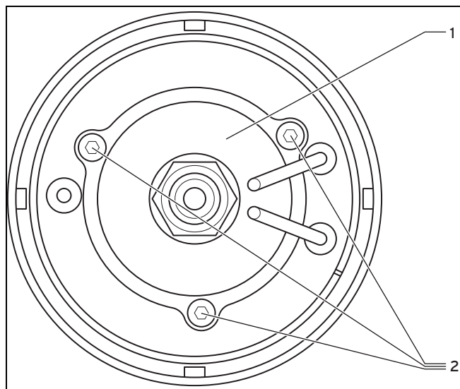
1 Luftdüse 2 Befestigungsschrauben
