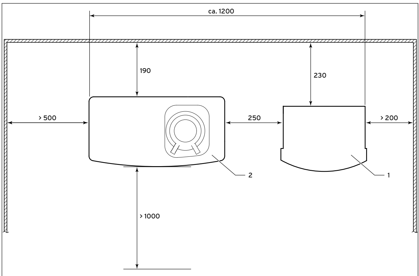
4.2 Abstände, Mindestabstände und Wartungsfreiräume für das mikro-BHKW
