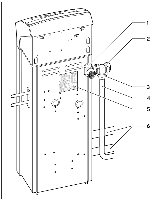
4.14 Rückansicht Wärmeauskopplungsmodul/Systemregler
