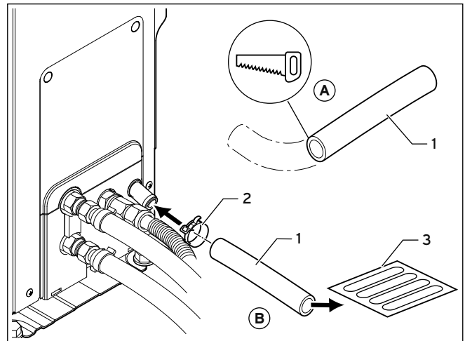
5.3 Kondenswasseranschluss ohne Kondenswasserpumpe
