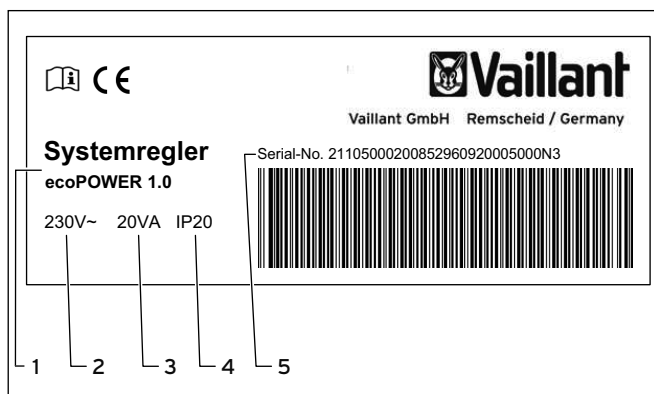
1.2 Typenschild Systemregler
