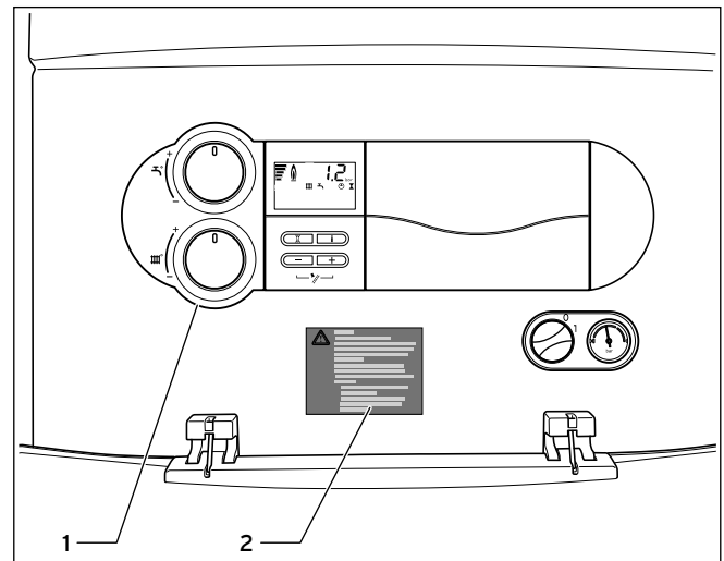
6.1 Aufkleber ecoTEC 0020109000
