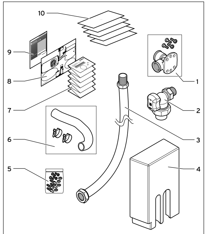
4.7 Lieferumfang Verpackungseinheit 5: Beipack Systeminstallation ecoPOWER 1.0
