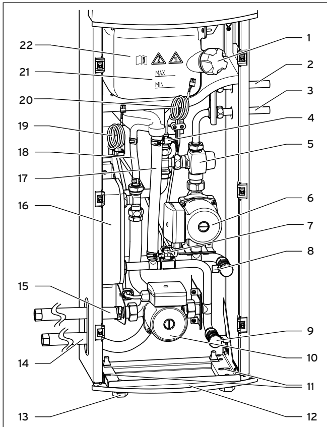
5.6 Wärmeauskopplungsmodul
