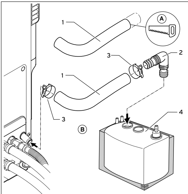
5.4 Kondenswasseranschluss mit Kondenswasserpumpe
