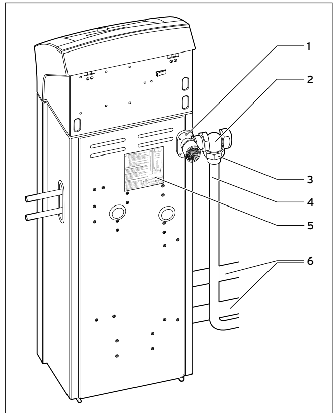
4.12 Rückansicht Wärmeauskopplungsmodul/Systemregler
