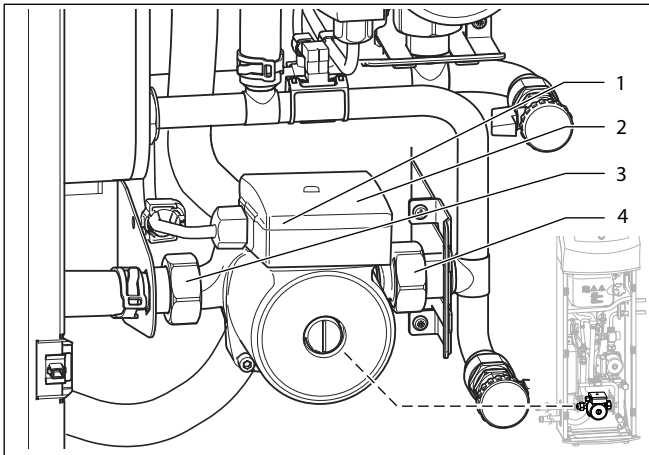
10.4 Kühlmittelpumpe
