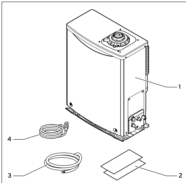
4.3 Lieferumfang Verpackungseinheit 1: KWK-Modul
