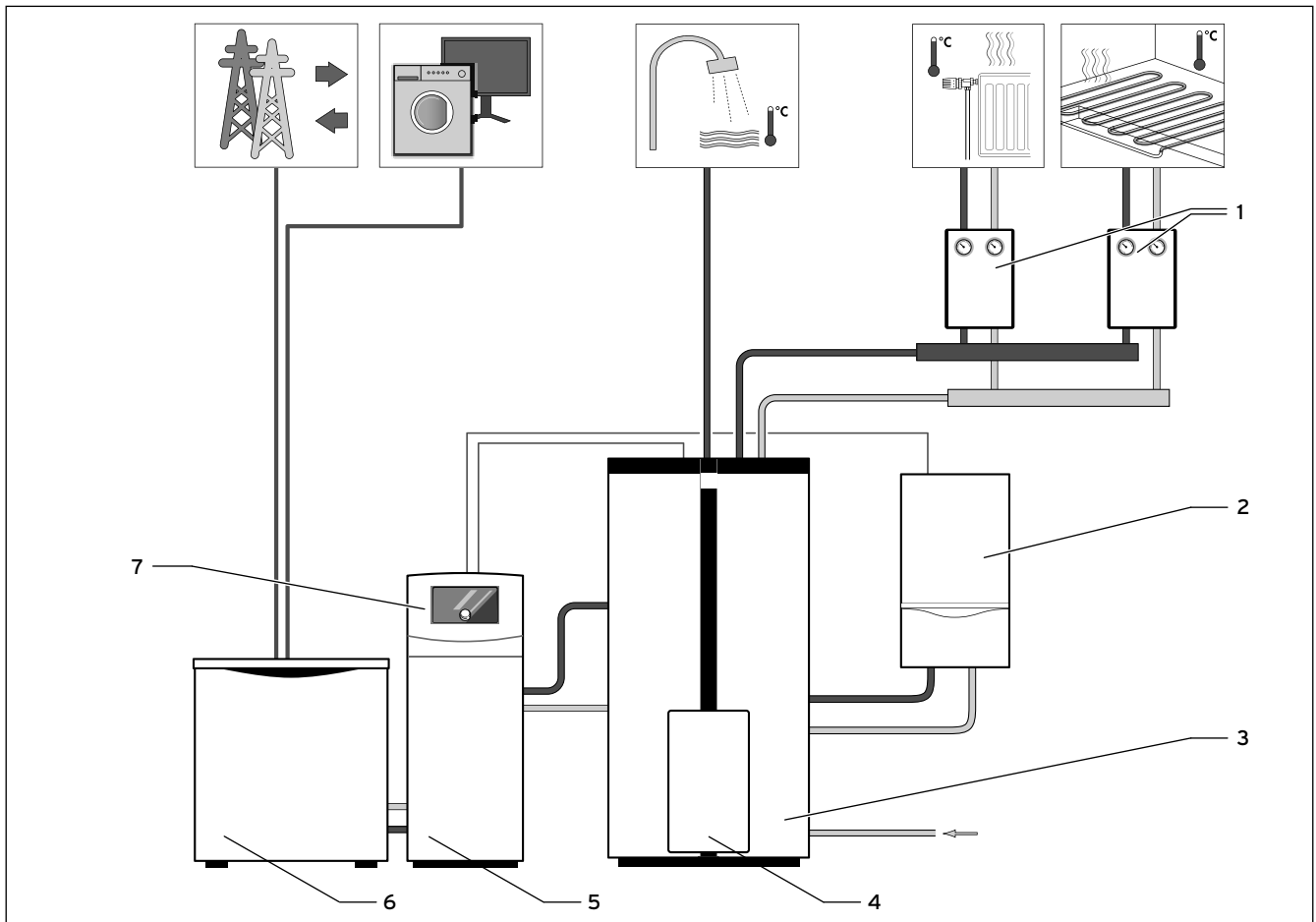
3.1 Prinzipdarstellung System ecoPOWER1.0
