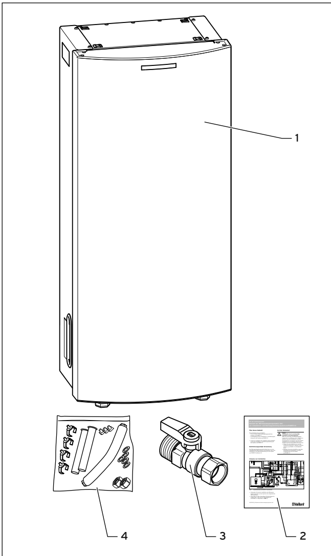
4.6 Lieferumfang Verpackungseinheit 4: Wärmeauskopplungsmodul
