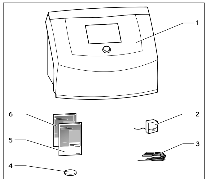
4.5 Lieferumfang Verpackungseinheit 3: Systemregler
