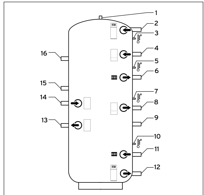
5.5 Pufferspeicher
