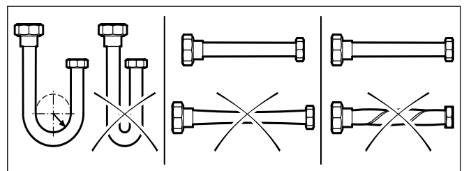
5.2 Hydraulikschläuche ausrichten
