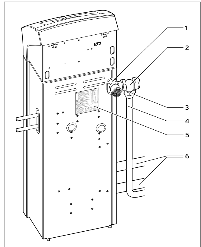
10.8 Rückansicht Wärmeauskopplungsmodul/Systemregler
