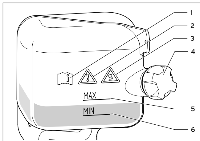
9.2 Kühlmittelbehälter
