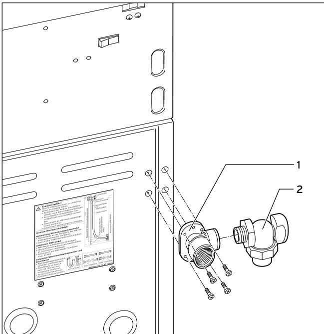
4.13 Wandscheibe und Gasabsperrhahn an das Wärmeauskopplungsmodul montieren
