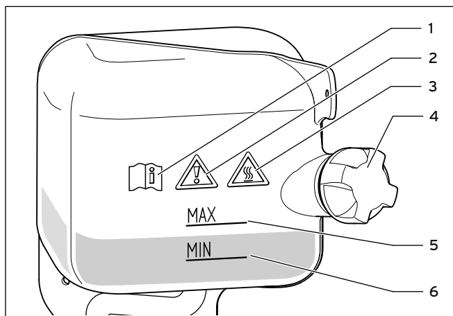
9.1 Kühlmittelbehälter
