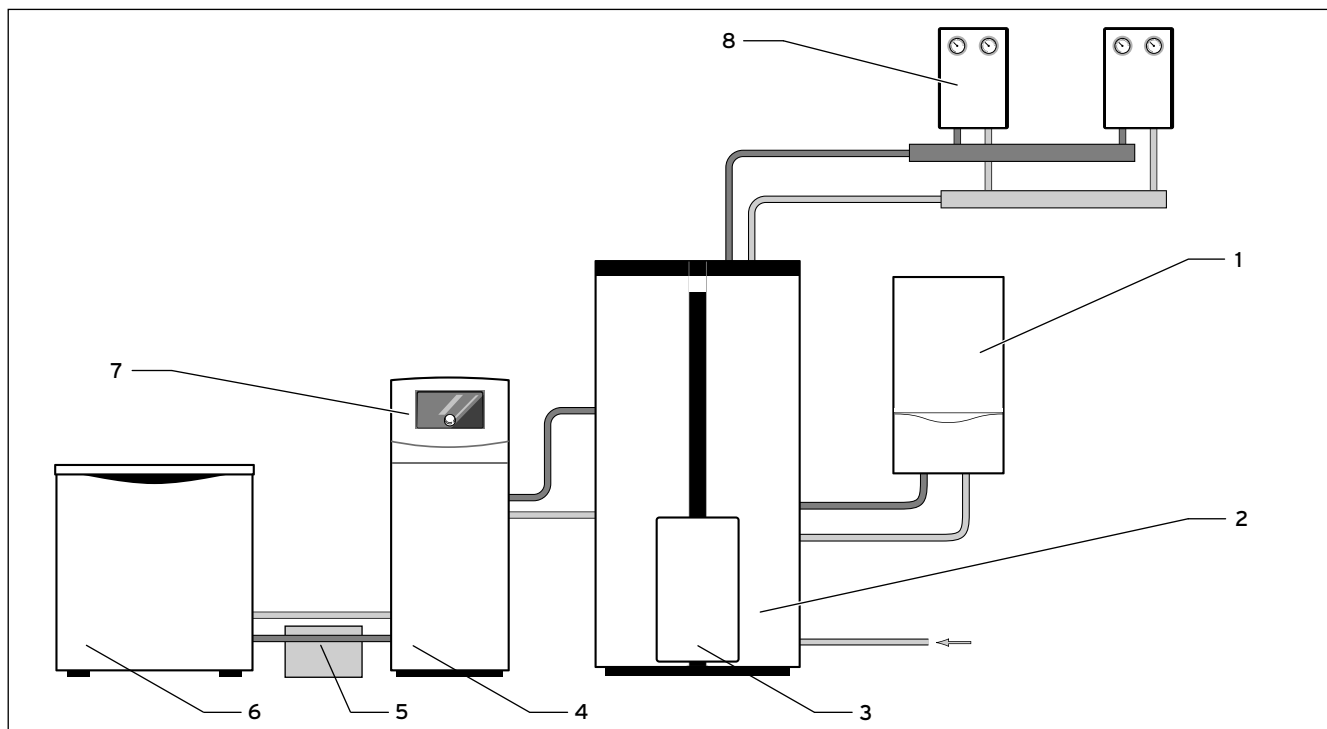
4.8 Anordnung der Systemkomponenten
