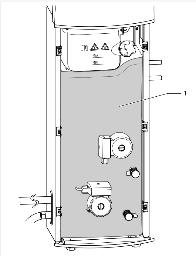
7.1 Wärmeauskopplungsmodul mit Front-Isoliermatte
