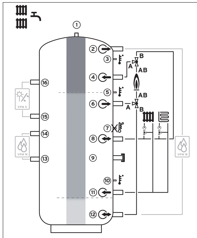
3.2 Pufferspeicher VPS/2: Beispiel für Anschluss Wohnbereich
