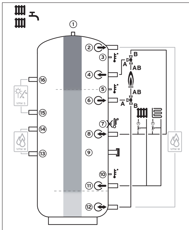
4.2 Anschlussschema Wohnanwendung
