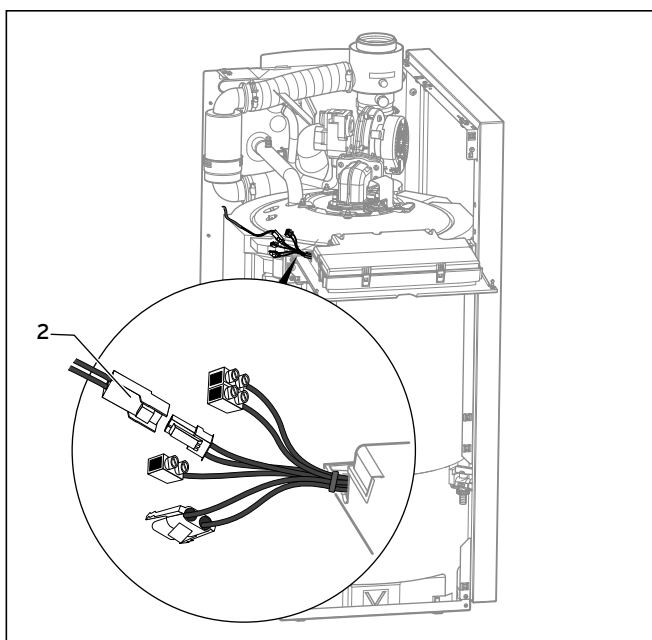
Abb. 5.6 Speichertemperaturfühler anschließen
