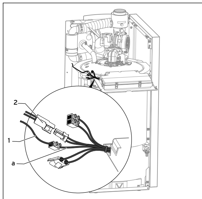
Abb. 5.5 Speicherfühler und Ladetemperaturfühler anschließen (actoSTOR)
