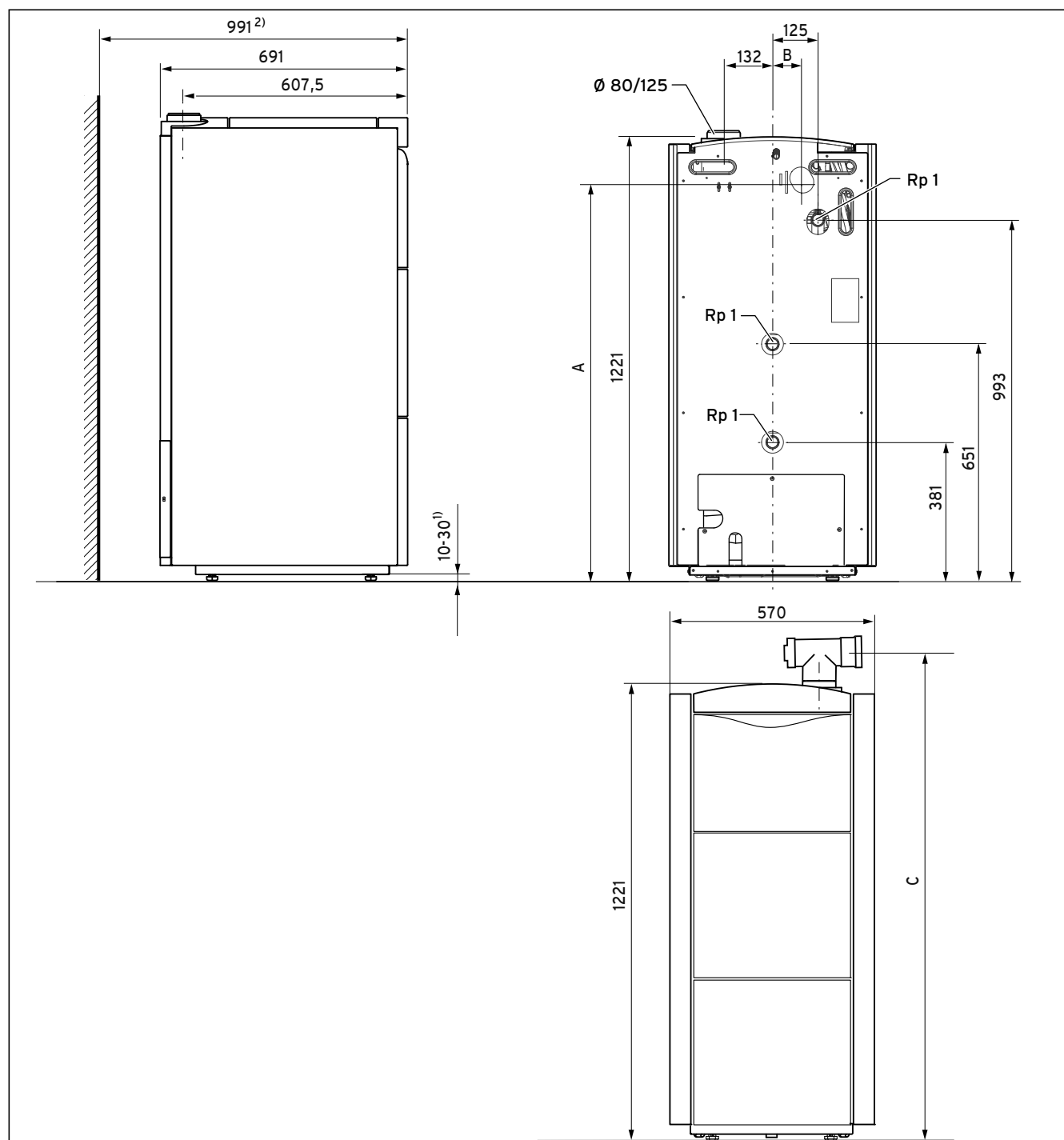
Abb. 4.2 Abmessungen
