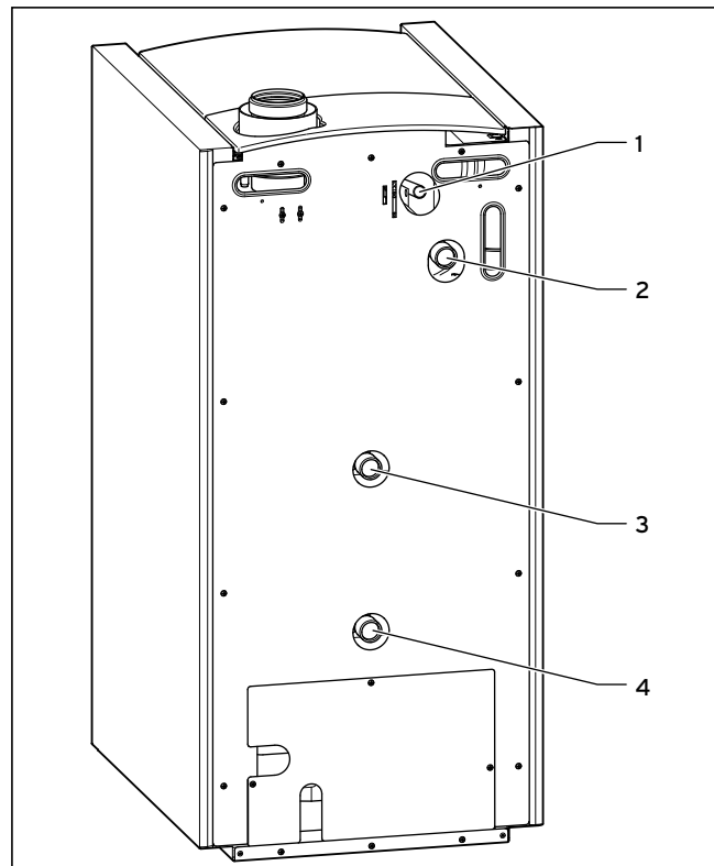
Abb. 5.4 Heizungsseitiger Anschluss
