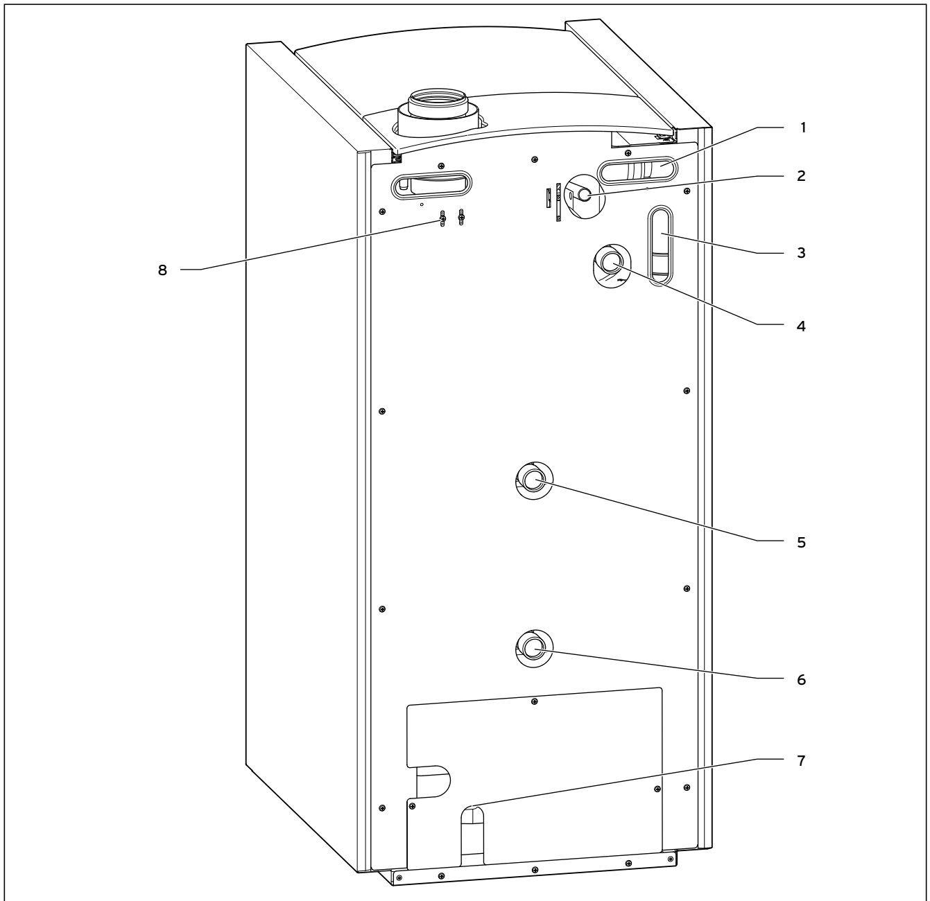
Abb. 3.2 Funktionselemente, Rückseite
