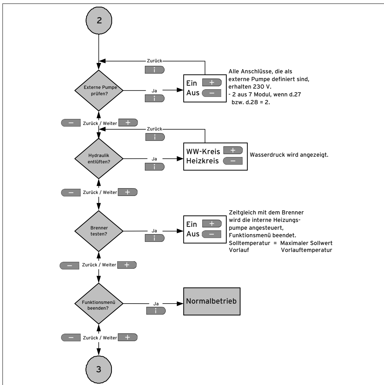
Abb. 6.1 Funktionsmenü (Fortsetzung)
