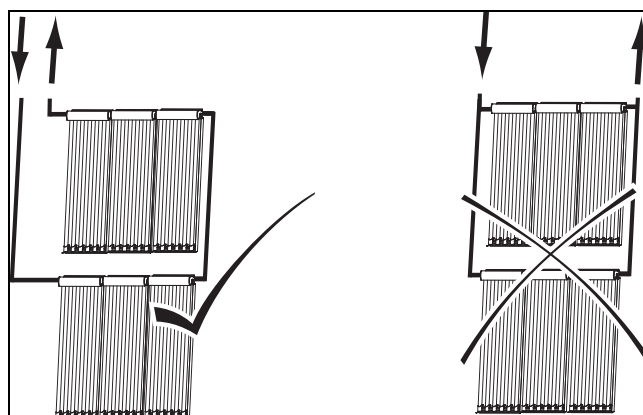
Abb. 5.4: Parallelverschaltung in Reihe übereinander (hier abgebildet: VTK 570/2)
