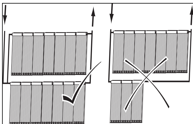
Abb. 5.6: Größe der Einzelreihen (hier abgebildet: VTK 570/2)
