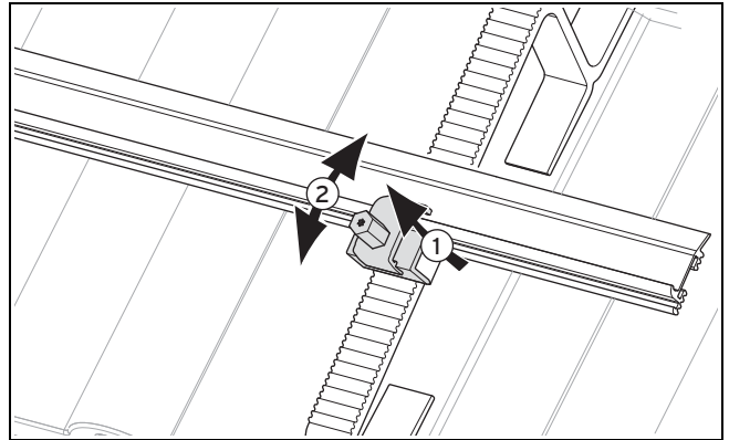
Abb. 4.32: Montageschienen austarieren
