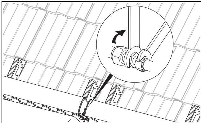
Abb. 4.38: Klemmringverbindung festziehen
