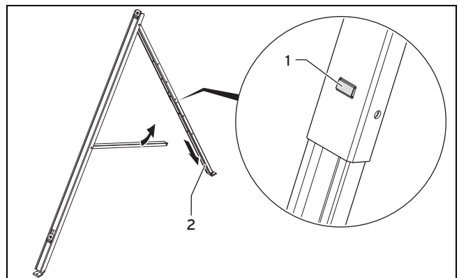
Abb. 5.14: Montagewinkel einstellen
