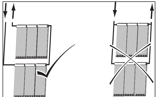
Abb. 4.4: Parallelverschaltung in Reihe übereinander (hier abgebildet: VTK 570/2)
