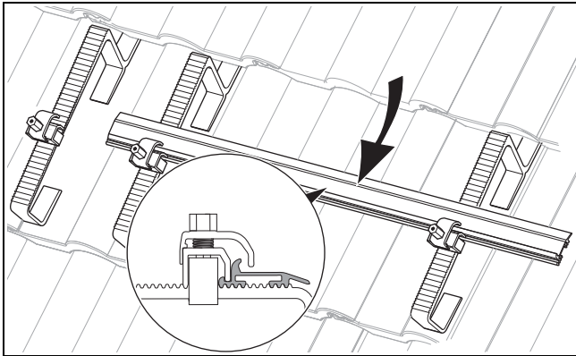
Abb. 4.30: Montageschienen montieren
