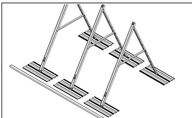
Abb. 5.22: Drei Gestelle ausgerichtet zur Aufnahme von zwei Kollektoren
