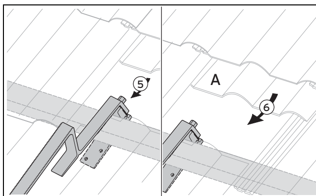
Abb. 4.22: Dachanker Typ P an der Dachlatte befestigen
