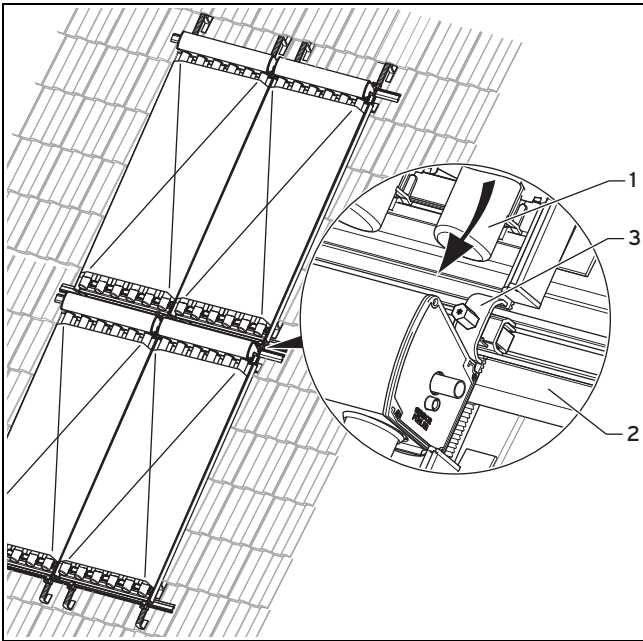
Abb. 4.41: Obere Kollektoren montieren
