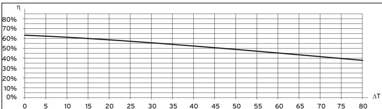
Abb. 10.3: Wirkungsgrad des VTK 570/2 und des VTK 1140/2 bei einer Einstrahlung EG von 300 W/m 2
