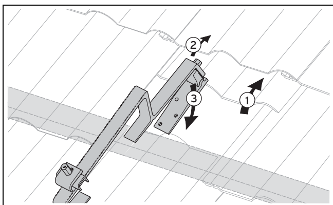
Abb. 4.20: Dachlatte freilegen und Dachanker Typ P anlegen
