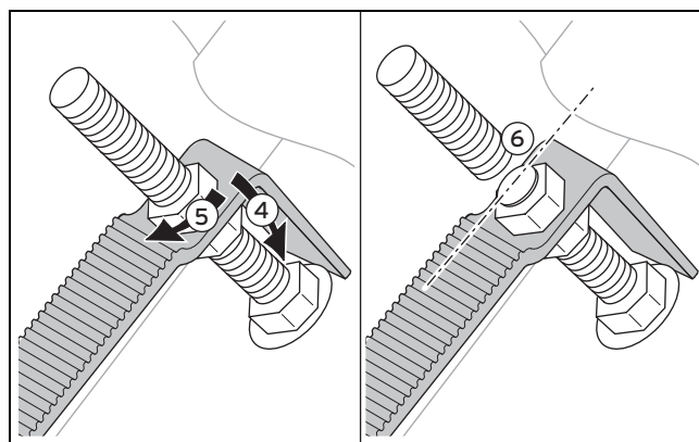
Abb. 4.29: Dachanker justieren, Gewindestange abschneiden
