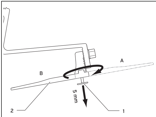
Abb. 4.16: Unterteil drehen
