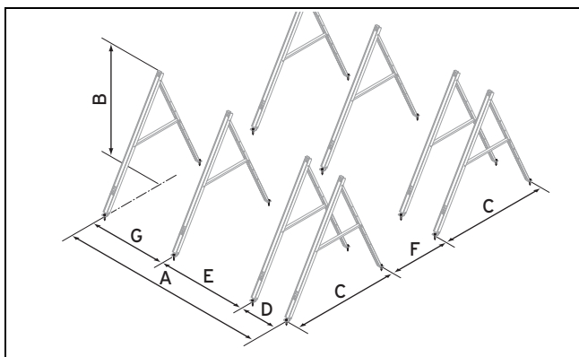
Abb. 5.11: Abstände der Gestelle VTK 570/2 und VTK 1140/2 in Kombination
