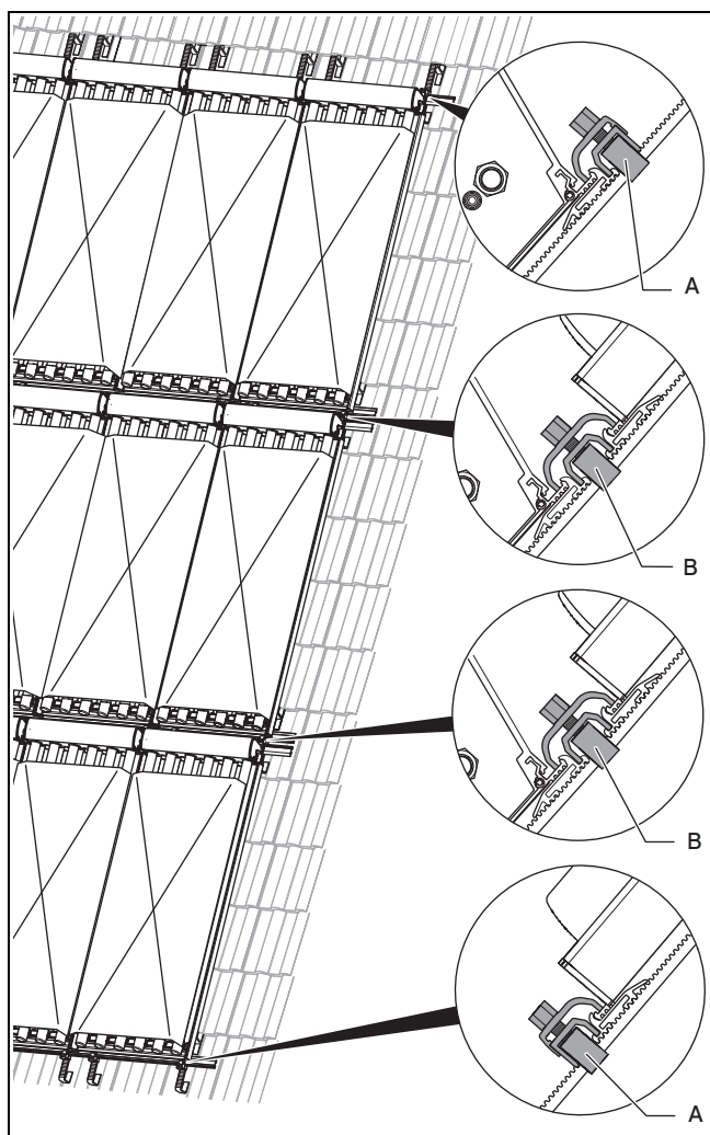
Abb. 4.10: Einbau-Set Aufdachmontage 3-reihig (hier: VTK 570/2)
