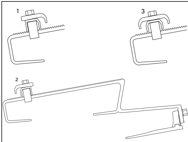
Abb. 4.15: Dachanker Typ P
