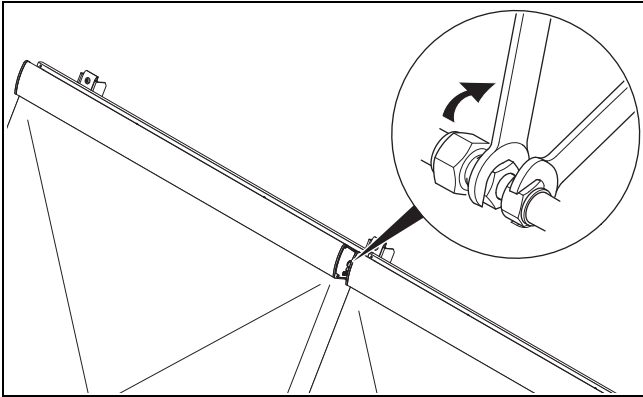
Abb. 5.37: Klemmringverbindung festziehen
