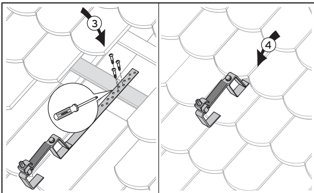
Abb. 4.24: Dachanker Typ S festschrauben und Schindeln wieder auflegen (hier dargestellt: an der Dachlatte)
