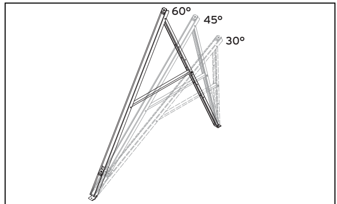
Abb. 5.13: Montagewinkel wählen
