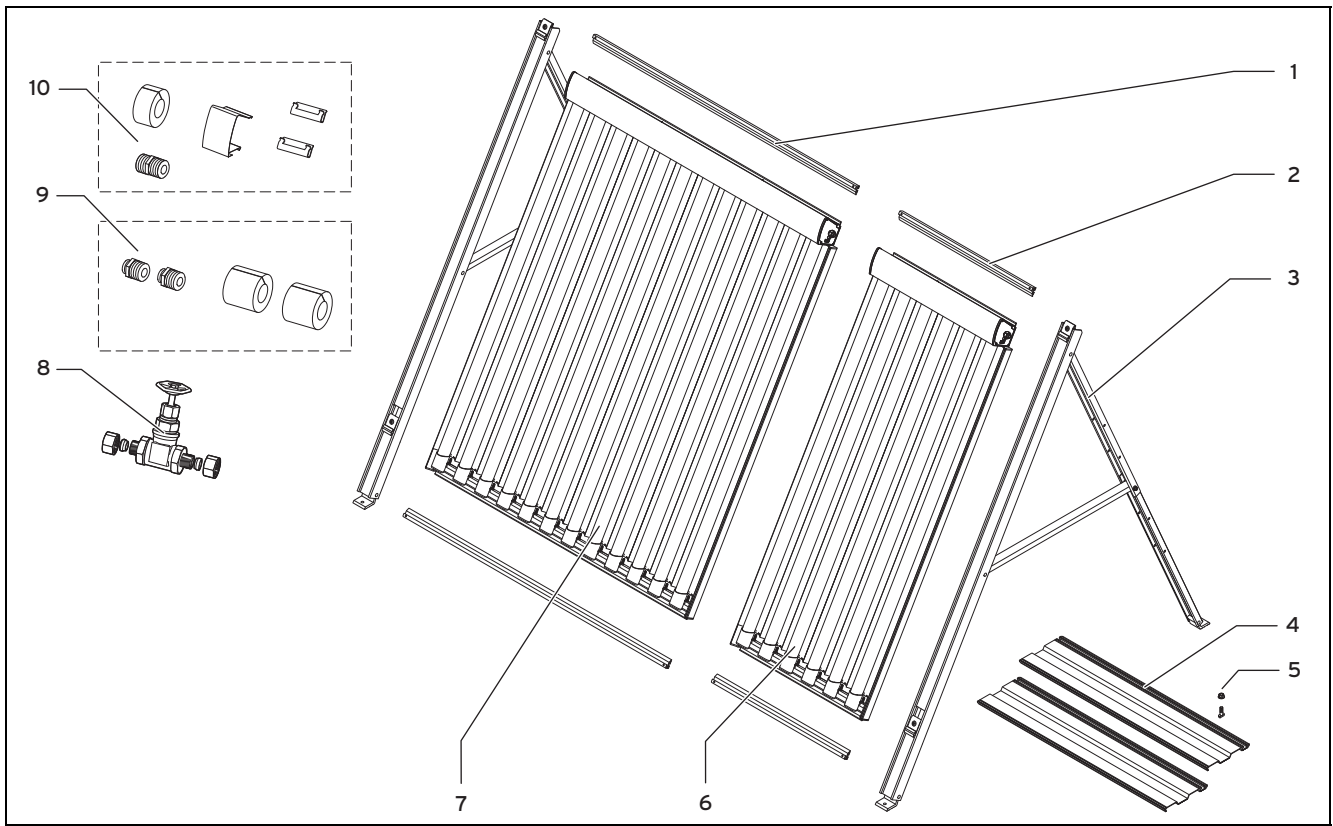
Abb. 5.1: Einbauset Flachdachmontage
