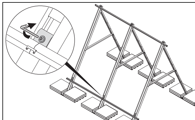
Abb. 5.30: Montageschienen unten befestigen
