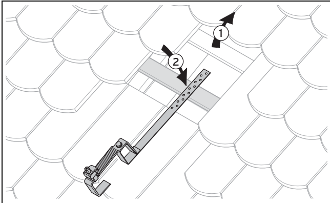
Abb. 4.23: Schindeln entfernen und Dachanker Typ S anlegen (hier dargestellt: an der Dachlatte)
