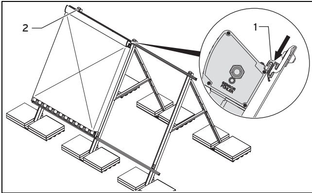
Abb. 5.32: Kollektor oben befestigen
