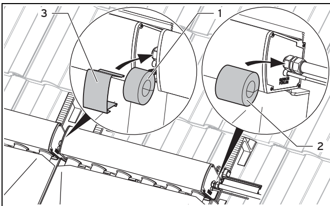
Abb. 4.43: Hydraulische Anschlüsse isolieren
