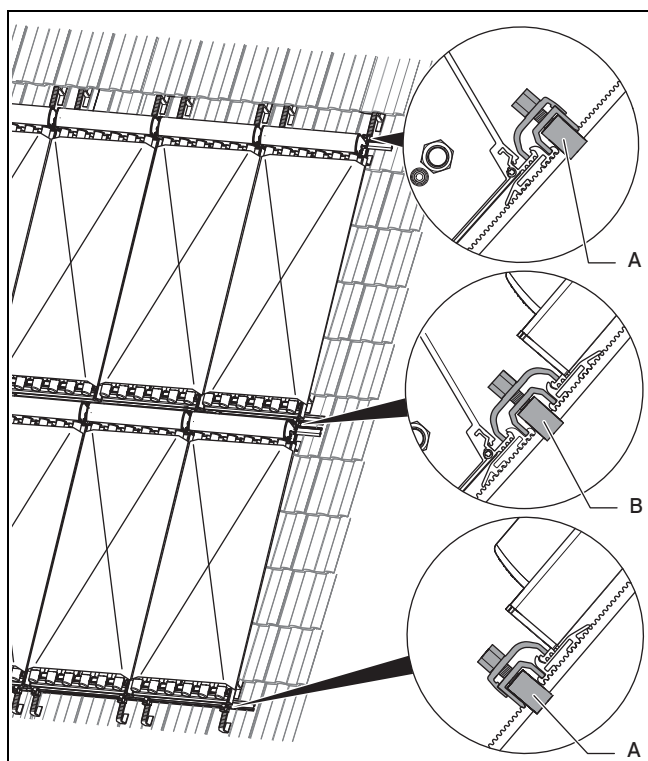
Abb. 4.9: Einbau-Set Aufdachmontage 2-reihig (hier: VTK 570/2)
