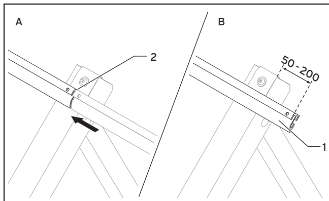
Abb. 5.28: Montageschienen an mehreren Gestellen anbringen
