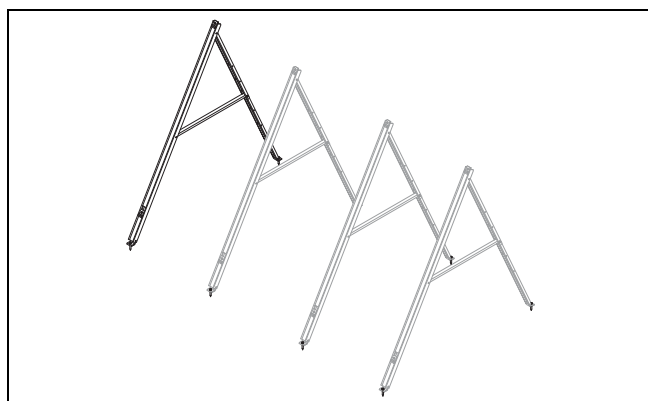
Abb. 5.16: Gestelle für Direktverschraubung
