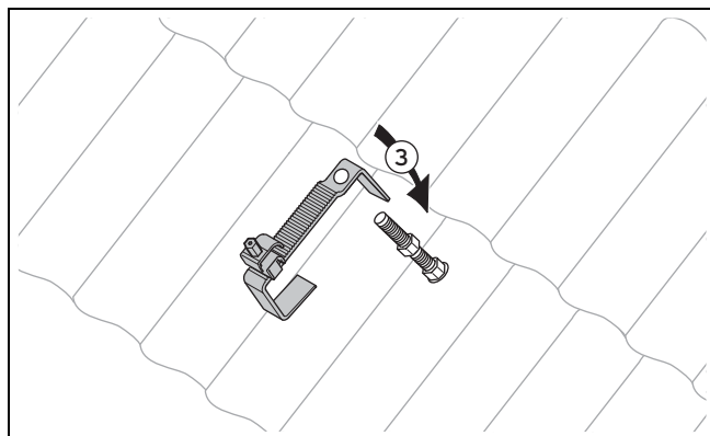
Abb. 4.28: Mutter festschrauben, Dachanker aufsetzen
