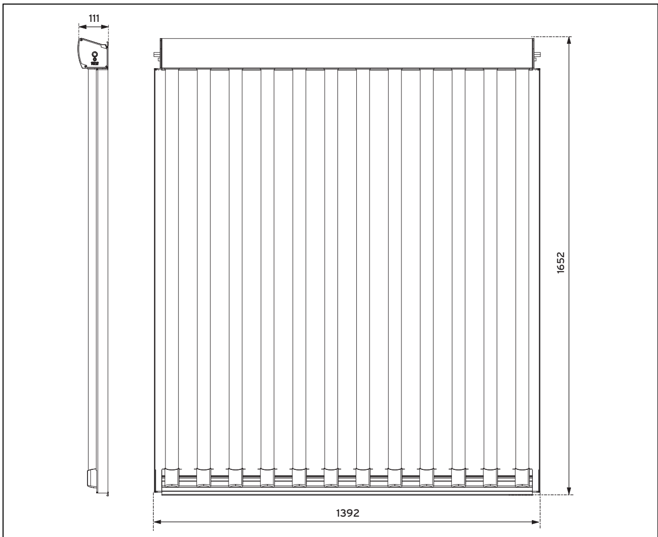
Abb. 10.2: Abmessungen VTK 1140/2
