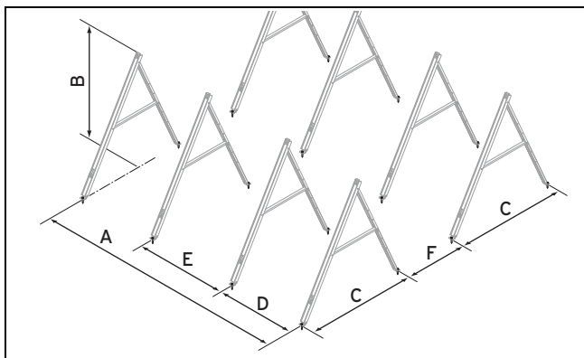
Abb. 5.10: Abstände der Gestelle 1140/2
