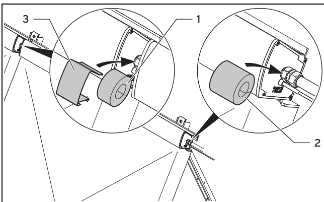
Abb. 5.39: Hydraulische Anschlüsse isolieren
