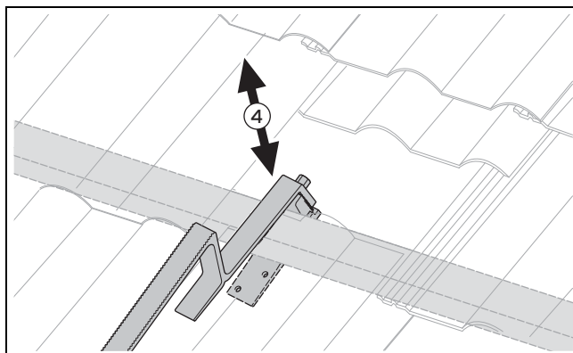
Abb. 4.21: Dachanker Typ P auf der Dachlatte korrekt positionieren
