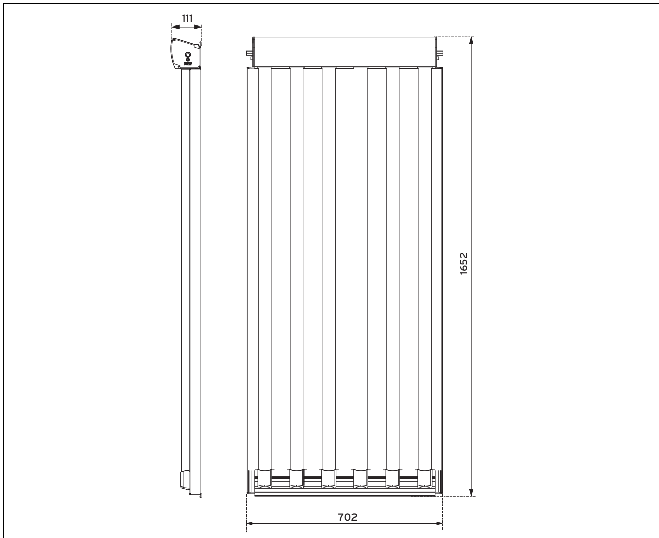
Abb. 10.1: Abmessungen VTK 570/2
