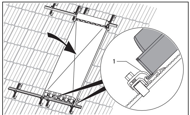
Abb. 4.33: Kollektor auflegen und einhaken
