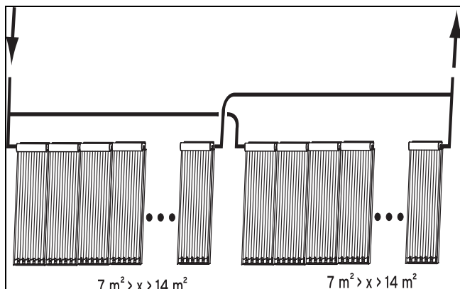
Abb. 5.5: Parallelverschaltung in mehreren Kollektorreihen (hier abgebildet: VTK 570/2)
