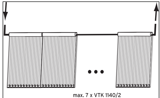
Abb. 4.3: Reihenschaltung VTK 1140/2
