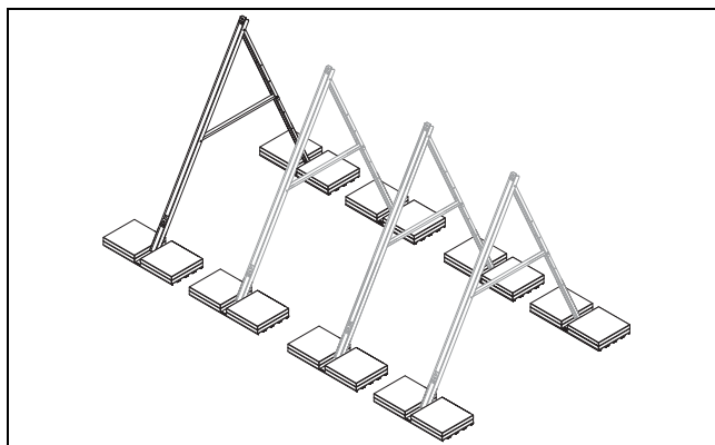
Abb. 5.17: Gestelle für Montage mit Beladungsplatten
