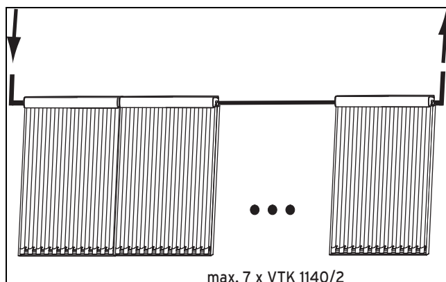
Abb. 5.3: Reihenschaltung VTK 1140/2
