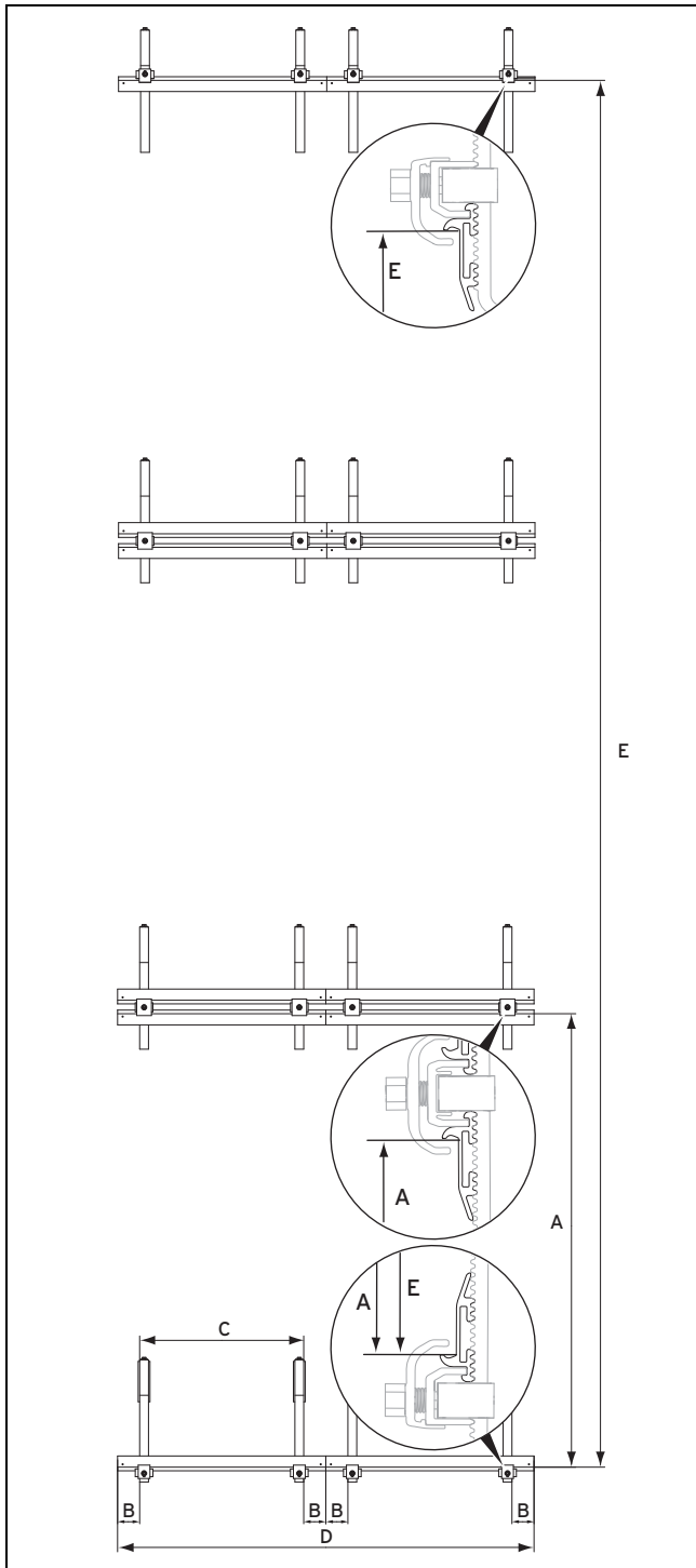
Abb. 4.14: Abstände bei Feldanordnung übereinander, 3-reihig
