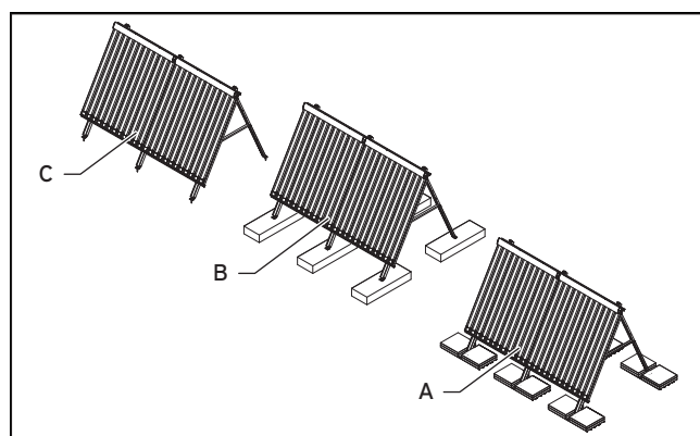
Abb. 5.7: Montagevarianten Flachdach
