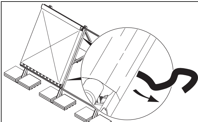
Abb. 5.33: Tragegurte entfernen
