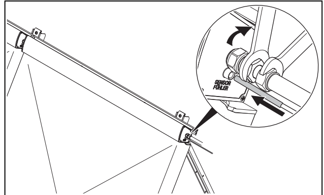
Abb. 5.38: Hydraulische Anschlüsse montieren
