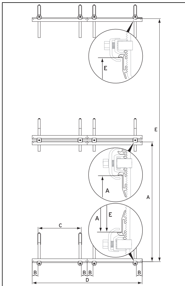
Abb. 4.13: Abstände bei Feldanordnung übereinander, 2-reihig
