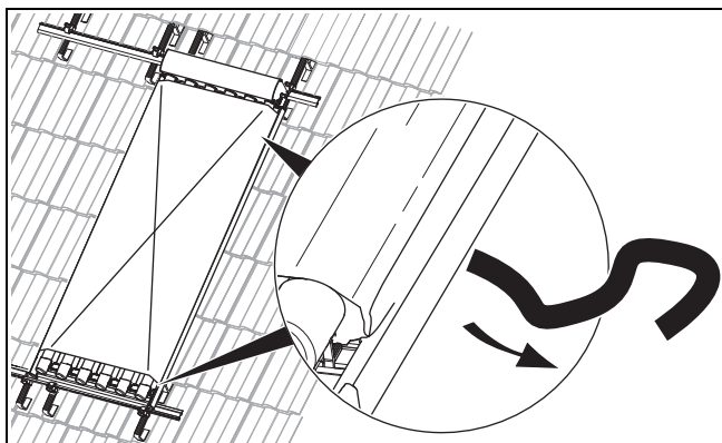
Abb. 4.35: Tragegurte entfernen
