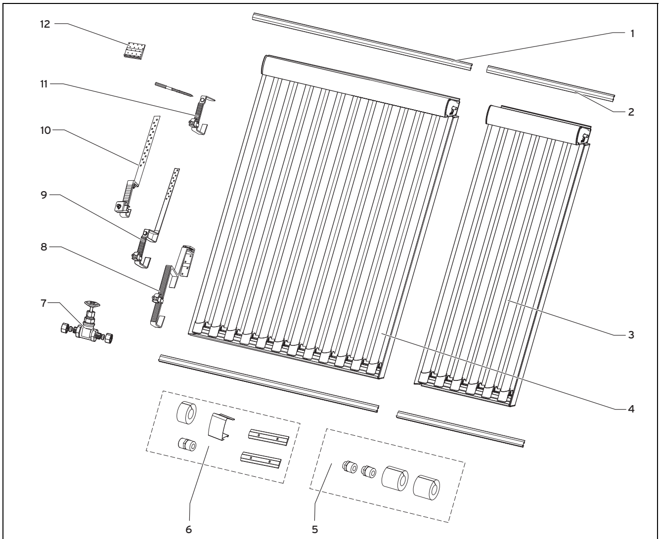
Abb. 4.1: Einbauset Aufdachmontage
