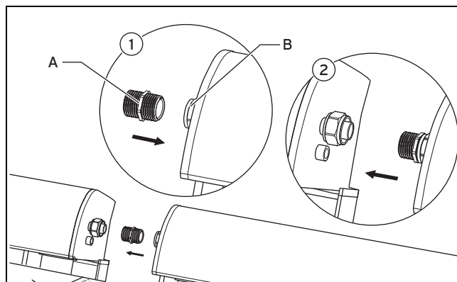
Abb. 4.37: Verbindungsstücke anbringen
