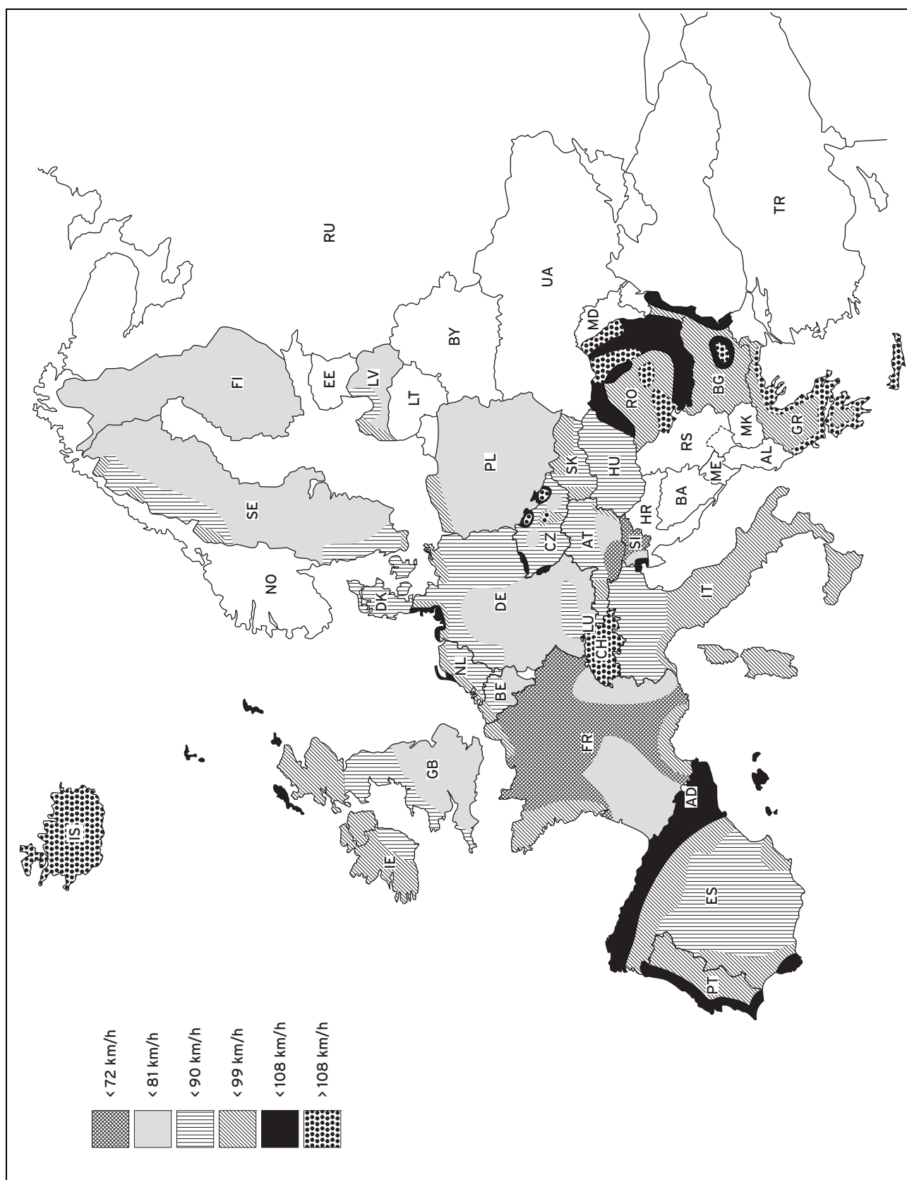
Abb. 5.8: Basiswindgeschwindigkeiten in Abhängigkeit vom Standort
