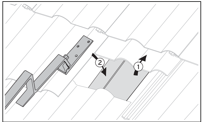
Abb. 4.17: Dachsparren freilegen und Dachanker Typ P anlegen
