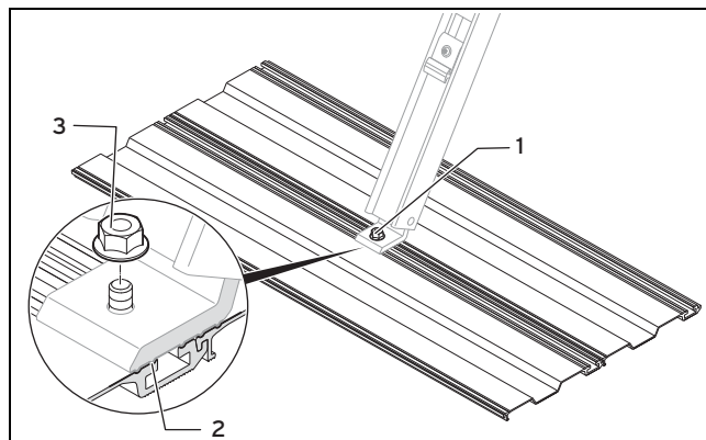
Abb. 5.20: Gestell auf Beladungsplatten verschrauben
