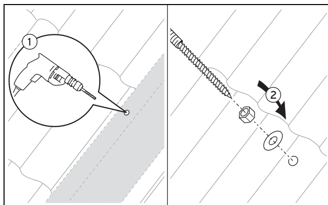
Abb. 4.27: Position des Dachankers auf dem Dachsparren festlegen
