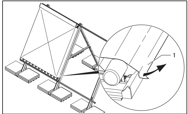
Abb. 5.34: Sonnenschutzfolie lösen
