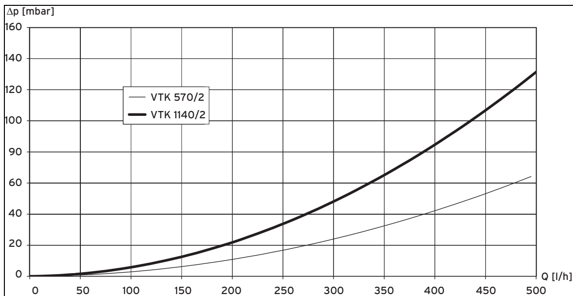
Abb. 10.5: Druckverlust
