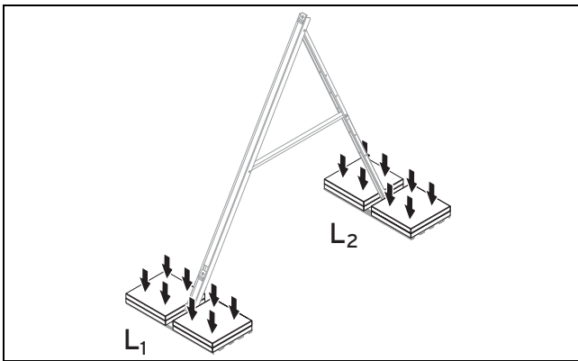
Abb. 5.9: Gewichte vorne (L 1 ) und hinten (L 2 )
