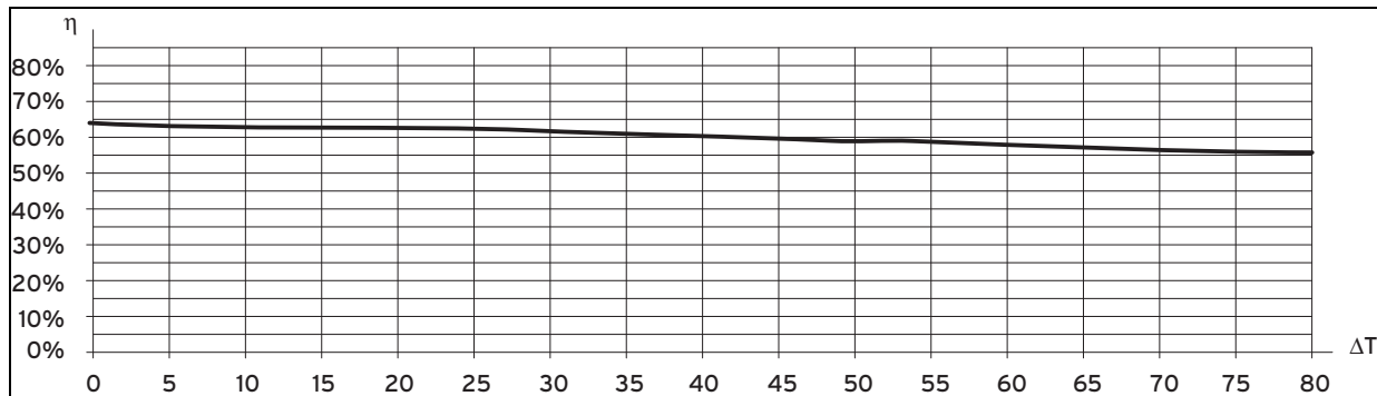
Abb. 10.4: Wirkungsgrad des VTK 570/2 und des VTK1140/2 bei einer Einstrahlung EG 800 W/m 2
