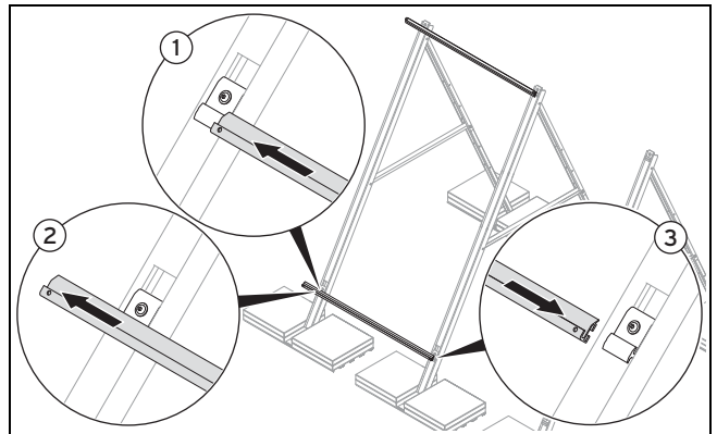
Abb. 5.27: Montageschienen aufschieben
