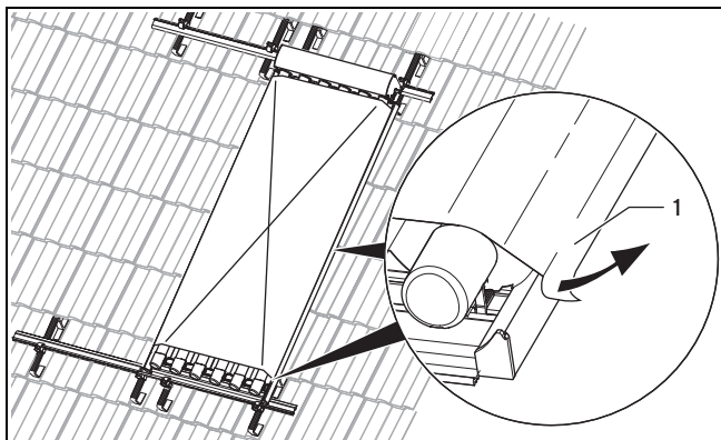
Abb. 4.34: Sonnenschutzfolie lösen
