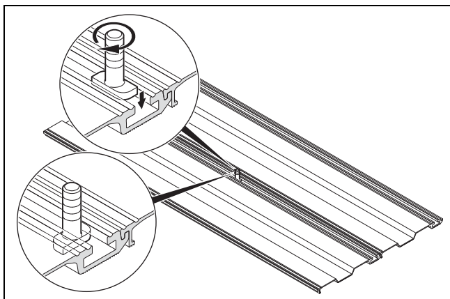
Abb. 5.19: Hammerkopfschraube einsetzen und fixieren
