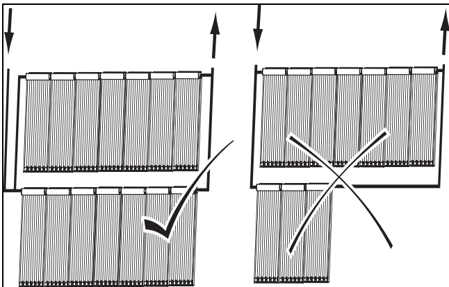
Abb. 4.6: Größe der Einzelreihen (hier abgebildet: VTK 570/2)
