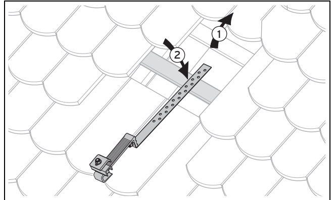
Abb. 4.25: Schindeln entfernen und Dachanker Typ S flach anlegen (hier dargestellt: an der Dachlatte)
