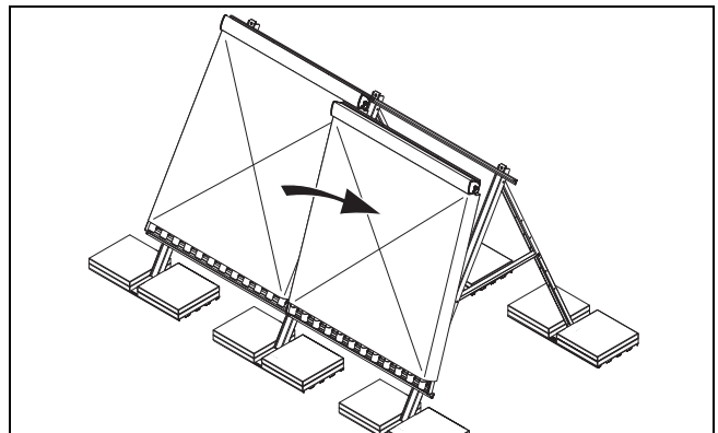
Abb. 5.35: Weiteren Kollektor montieren
