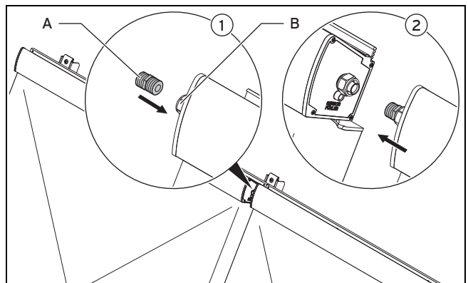
Abb. 5.36: Verbindungsstücke anbringen
