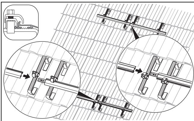
Abb. 4.31: Montageschienen verbinden
