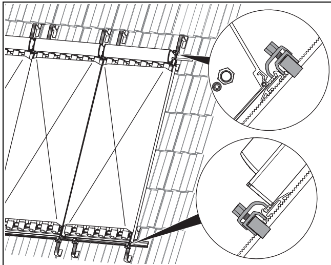
Abb. 4.8: Einbau-Set Aufdachmontage 1-reihig (hier: VTK 570/2)
