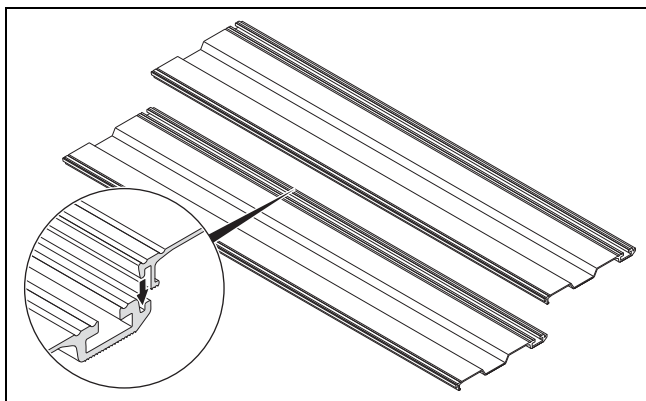
Abb. 5.18: Zwei Beladungsplatten verbinden
