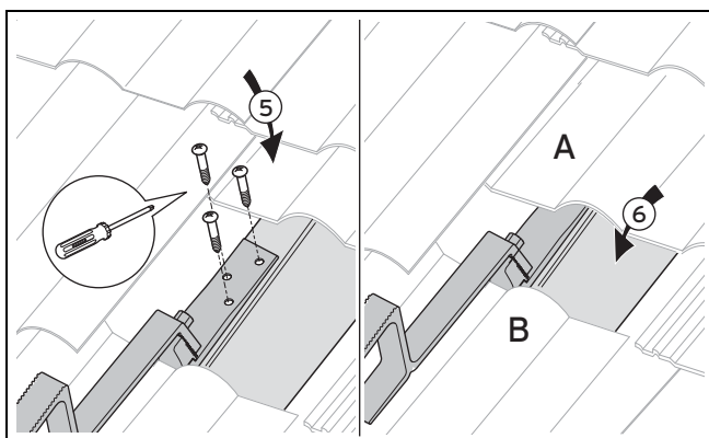
Abb. 4.19: Dachanker Typ P auf dem Dachsparren befestigen
