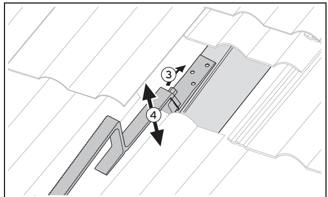
Abb. 4.18: Dachanker Typ P auf dem Dachsparren korrekt positionieren
