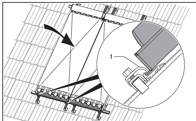
Abb. 4.36: Weiteren Kollektor montieren
