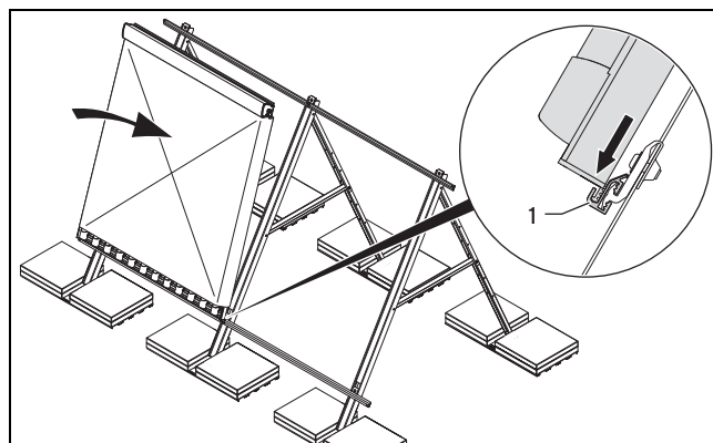
Abb. 5.31: Kollektor unten einhaken
