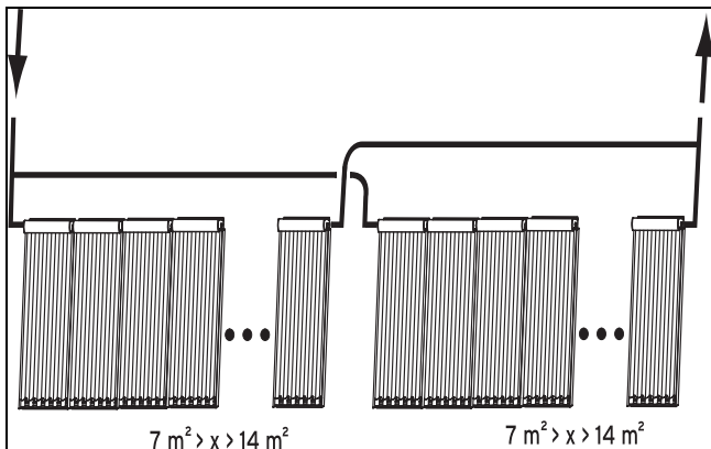
Abb. 4.5: Parallelverschaltung in mehreren Kollektorreihen (hier abgebildet: VTK 570/2)
