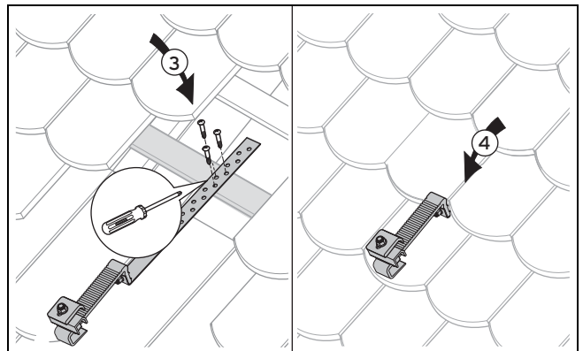
Abb. 4.26: Dachanker Typ S flach festschrauben und Schindeln wieder auflegen (hier dargestellt: an der Dachlatte)
