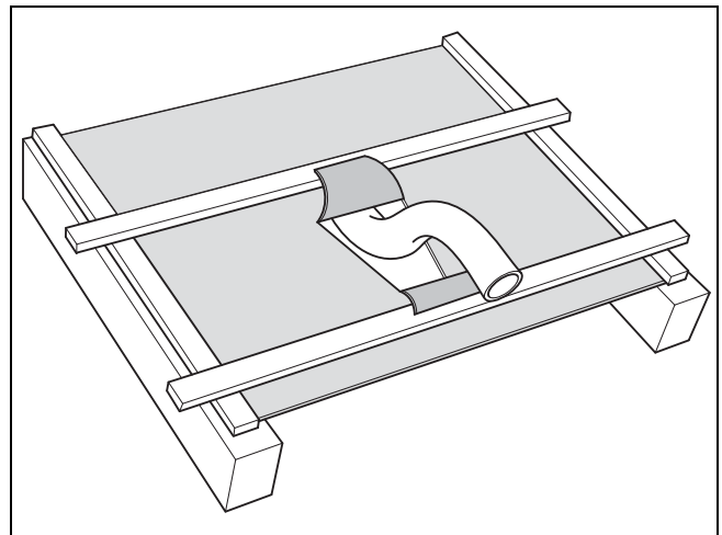
Abb. 4.7: Rohr durch Unterspannbahn führen
