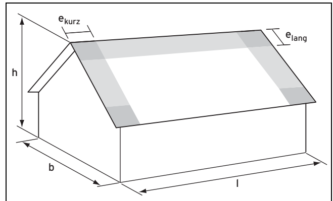
Abb. 4.11: Randabstände e_{\text{kurz}} und e_{\text{lang}}
