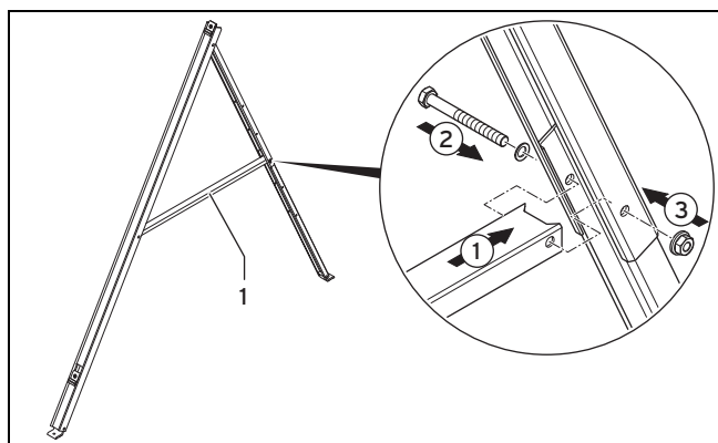
Abb. 5.15: Traverse in der Teleskopschiene fixieren
