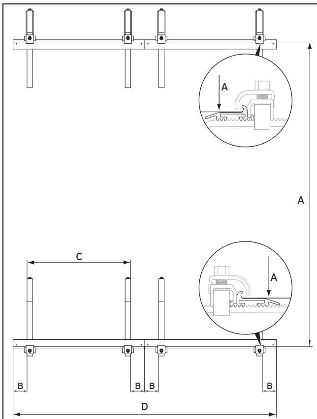
Abb. 4.12: Abstände bei Feldanordnung nebeneinander
