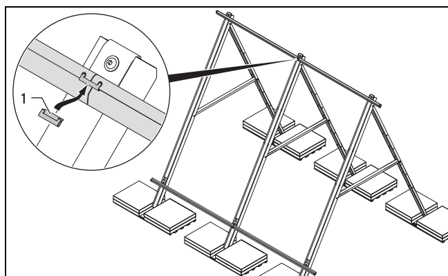
Abb. 5.29: Montageschienen verbinden
