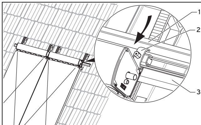
Abb. 4.40: Mittlere Montageschiene positionieren
