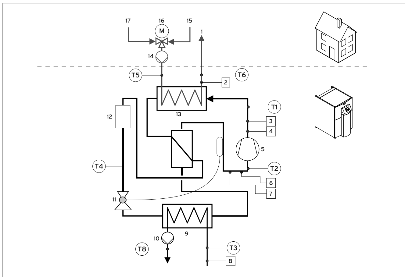
17.1 Anhang, Wärmepumpenschema VWS ..0/2
