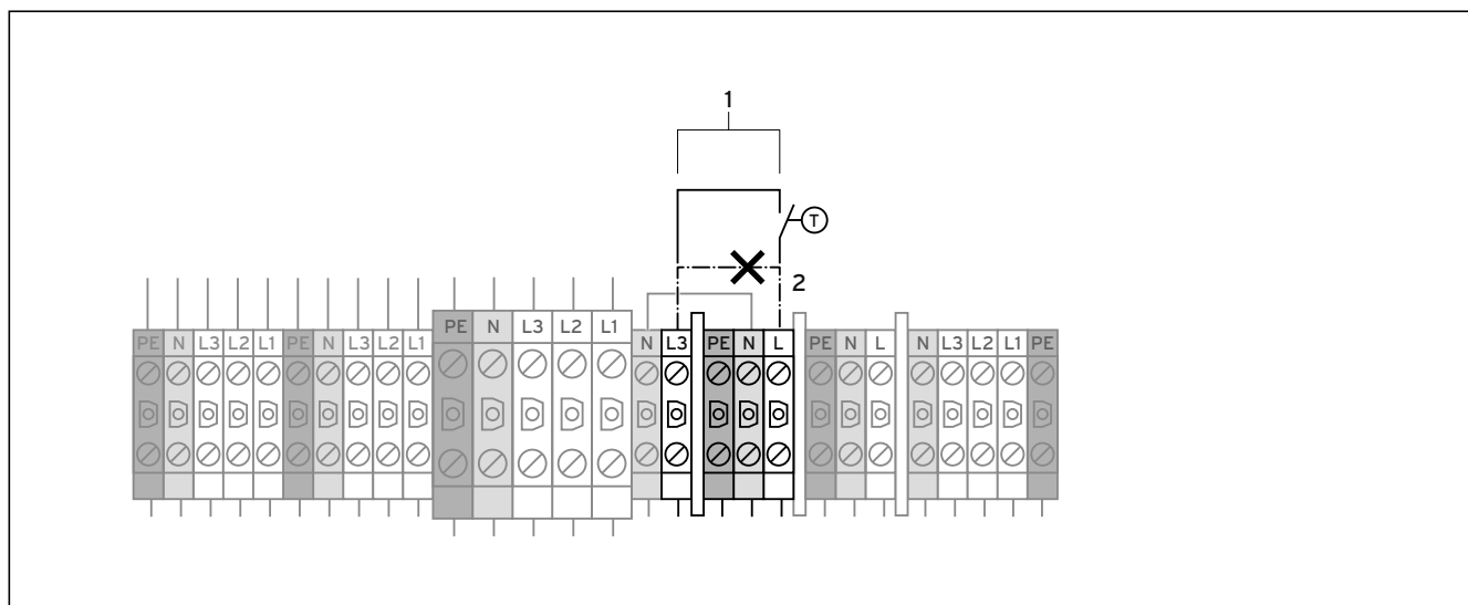
7.13 Maximalthermostat anschließen VWW
