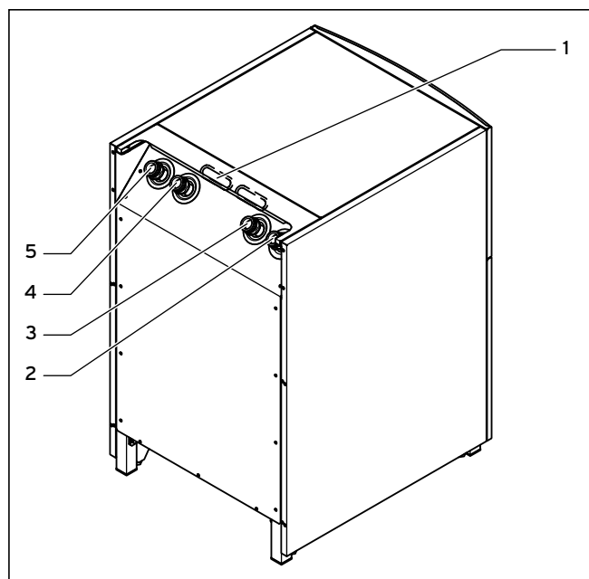
3.4 Rückansicht
