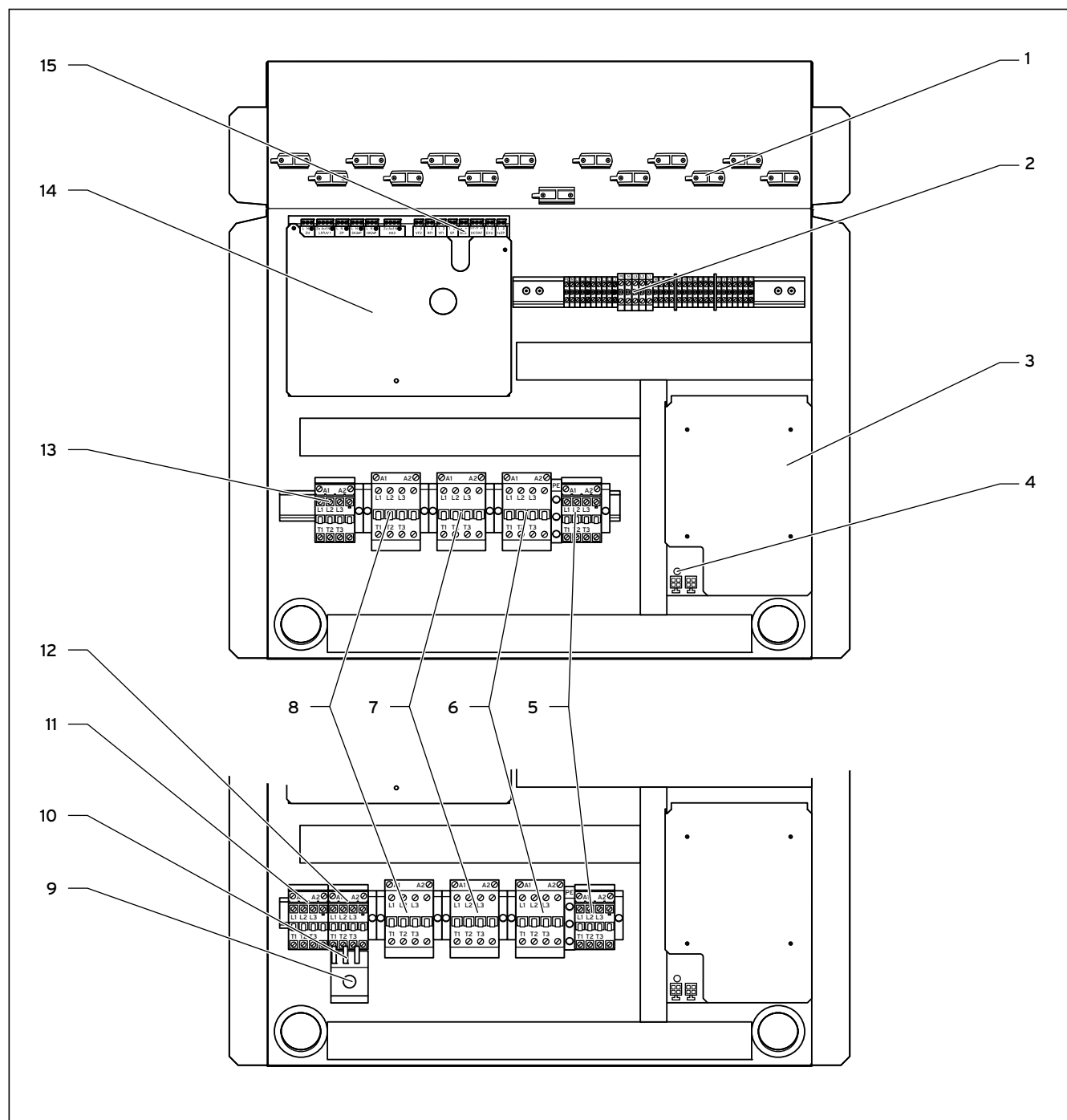
7.1 Elektro-Schaltkasten VWS und VWW 220/2 - 300/2
