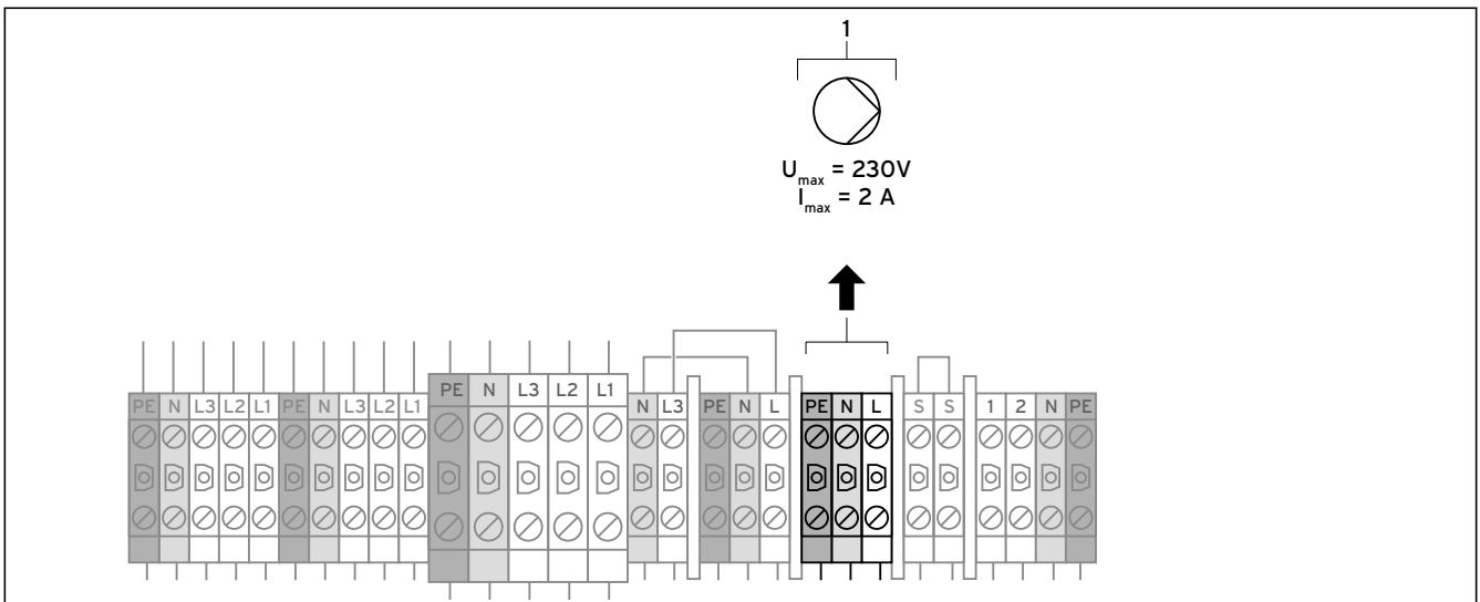
7.7 Externe Heizkreispumpe anschließen VWS
