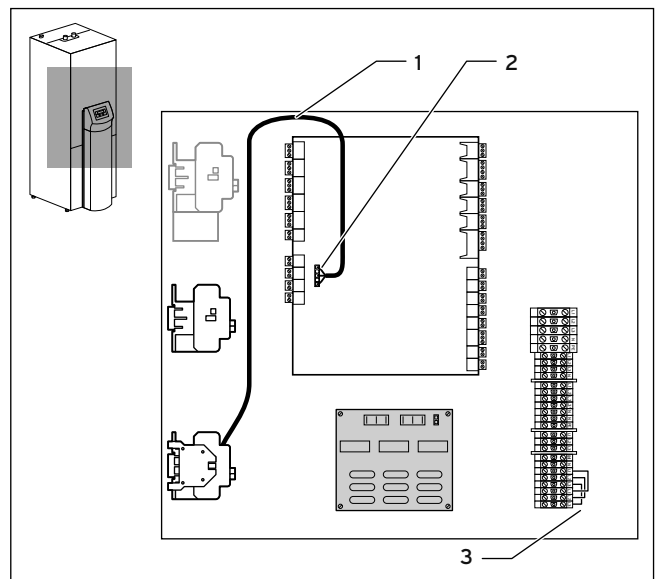
Kuva 4.8 Kompressorin vaiheentarkkailun purkamisen VWS/VWW/VWL-S ..2 und VWS ..3
