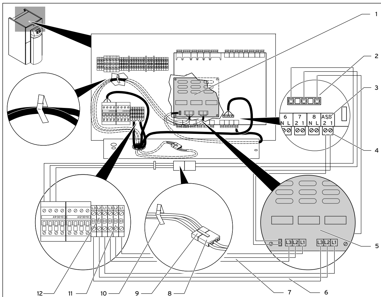
Fig. 4.6 Tilslutning af monteringsskiner til geoTHERM VWS/VWW/VWL-S ..1 og VWS ..4
