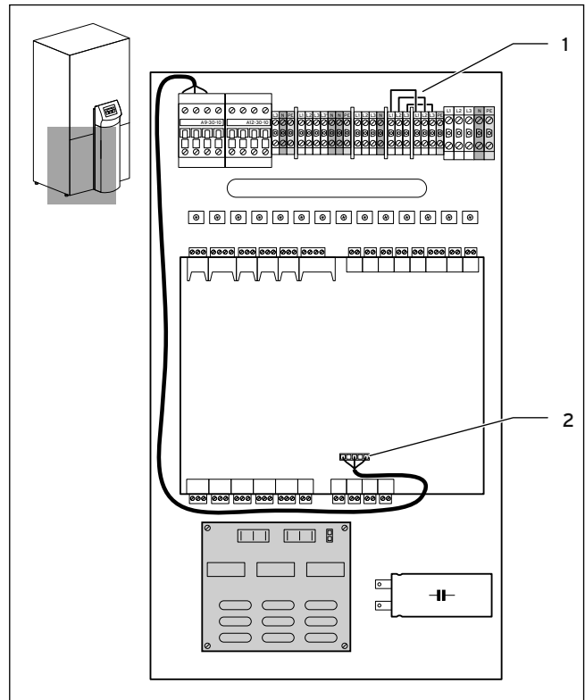
Kuva 4.2 Kompressorin vaiheentarkkailun purkaminen geoTHERM VWL
