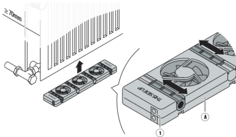
Abb. 1 - Position des SpeedComfort (A).
