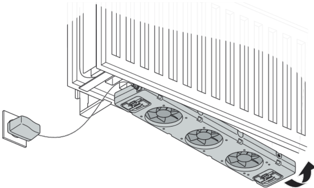
Abb. 2 - Anbringen des SpeedComfort (A).
