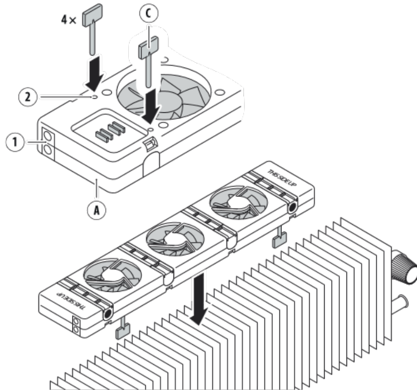
Abb. 8 - Anbringen eines Fußes (C).
