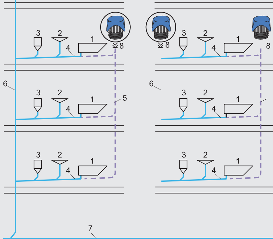
Be- und Entlüftung über Dach
