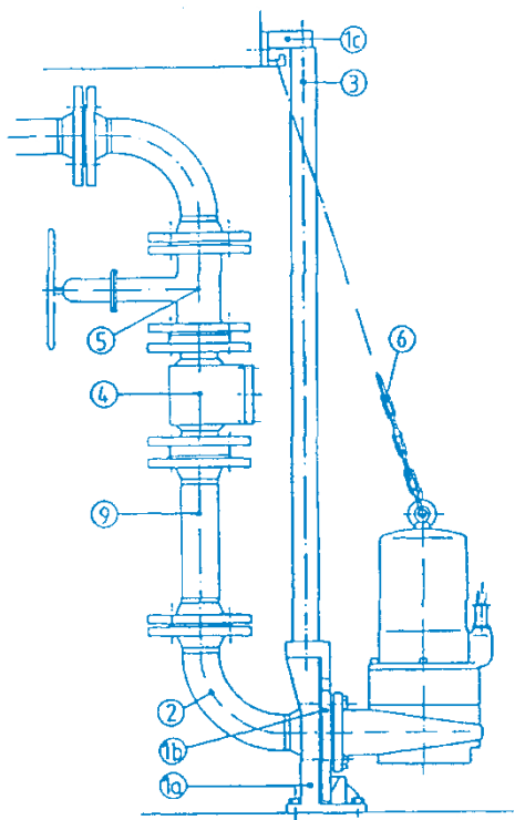
Montagem do poço com tubo condutor
