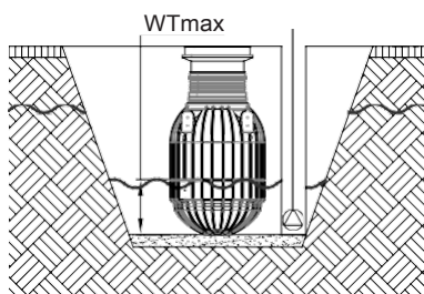
Tankserie SUF 2-200-2 / SUF 4-500
