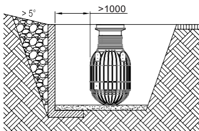
Tankserie SUF 2-200-2 / SUF 4-500
