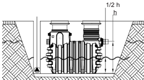
Tankserie SUF 7-700 / SUF 15-1500 / SUF 15-1500
