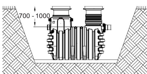
Tankserie SUF 7-700 / SUF 15-1500 / SUF 15-1500
