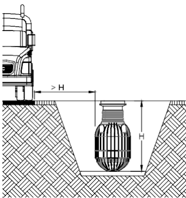
Tankserie SUF 2-200-2 / SUF 4-500
