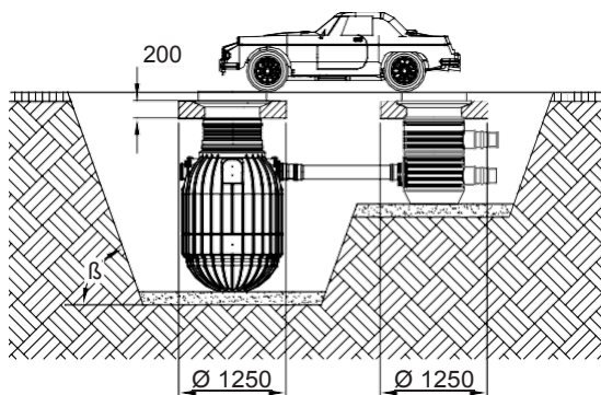
Tankserie SUF 2-200-2 / SUF 4-500
