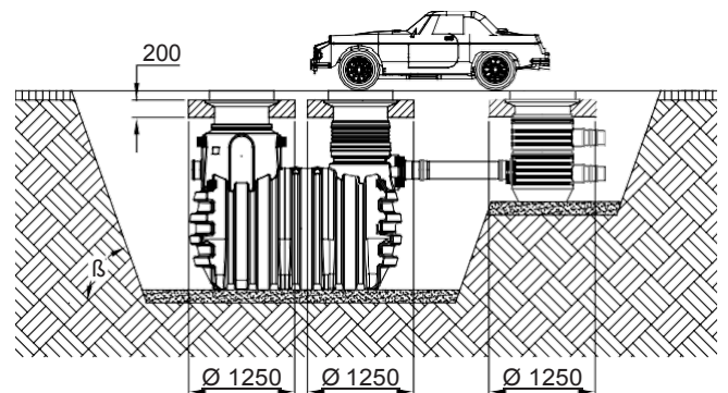
Tankserie SUF 7-700 / SUF 15-1500 / SUF 15-1500
