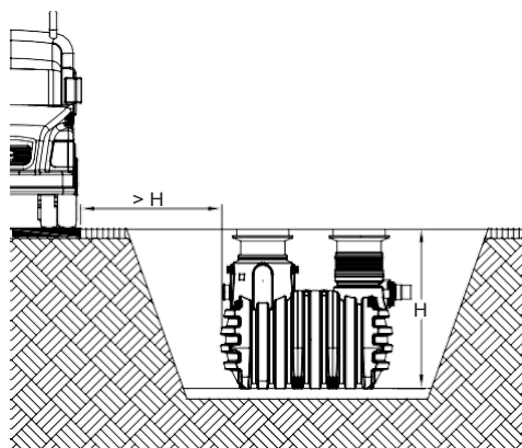
Tankserie SUF 7-700 / SUF 15-1500 / SUF 15-1500
