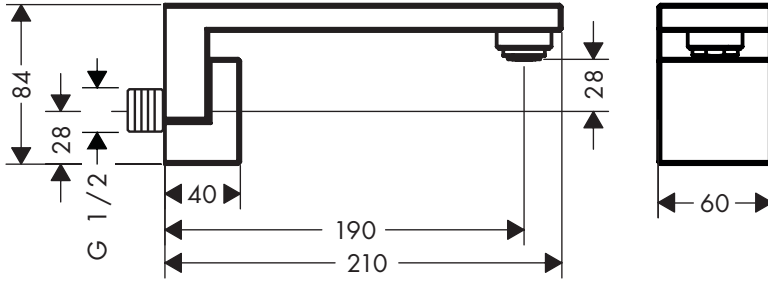
AXOR Edge 46410000 / 46411000
