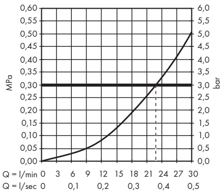
AXOR Edge 46410000 / 46411000
