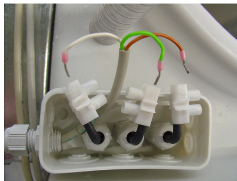
Collegamento sensori livello di riempimento
