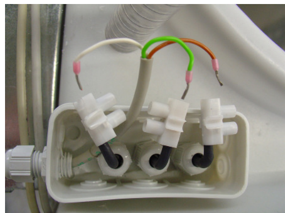
Anschluss Füllstandssensoren
