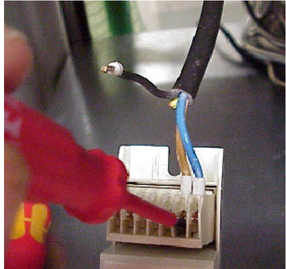
Leitungen trennen/anschiessen
