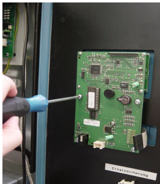
Svitare le viti di fissaggio
