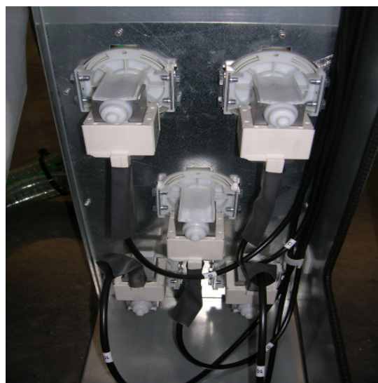
Raccord électrique de la pompe à sédiments
