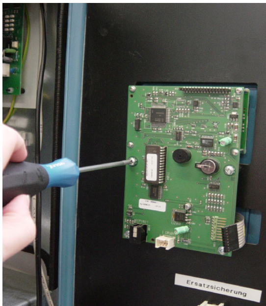
Desserrer les vis de fixation
