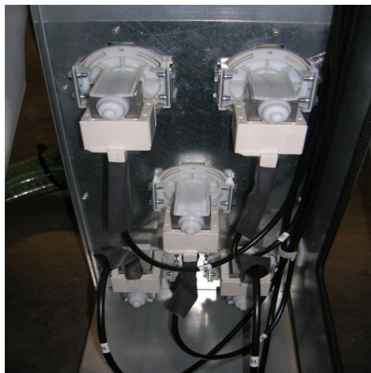
collegamento alla corrente della pompa di sedimentazione
