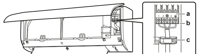
a Klemmleiste b Block für elektrische Komponenten c Kabelschelle
