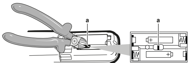
a Adressierungs-Jumper
