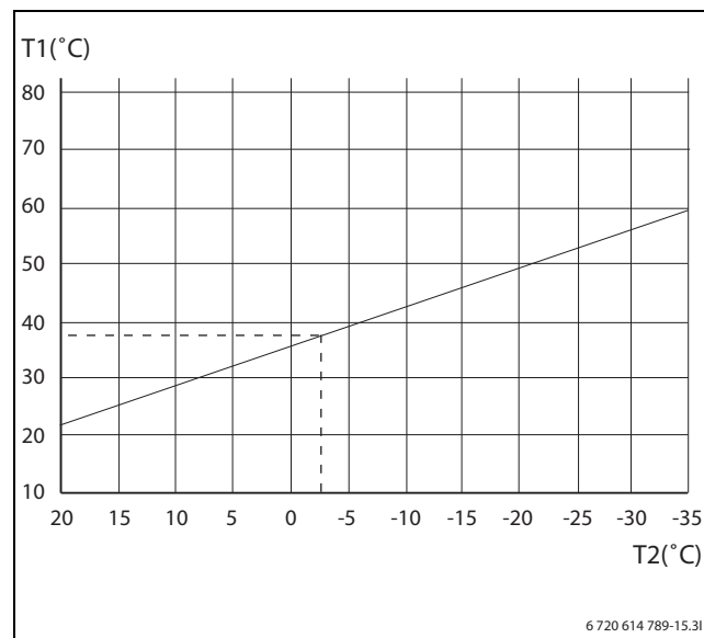
Bild 22 Heizkörper
