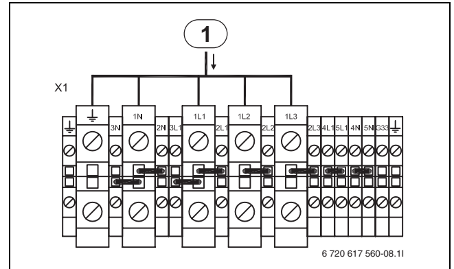
Bild 39 Standardausführung, STE 130-1 - 170-1
