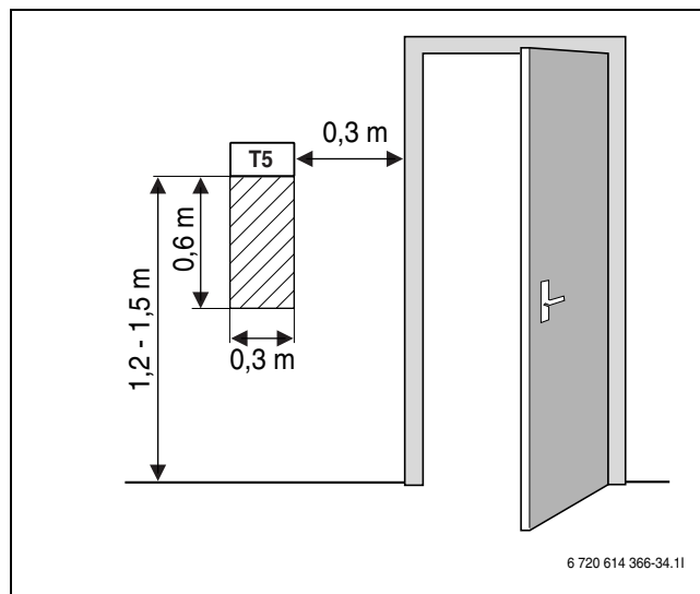
Bild 20 Empfohlener Montageplatz für Raumtemperaturfühler T5
