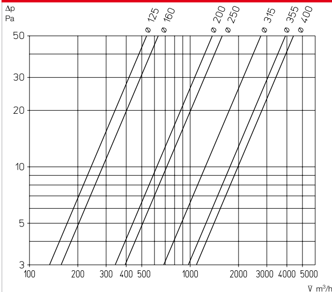
Kennlinien Druckverlust DDF bei Ablufteinsatz
