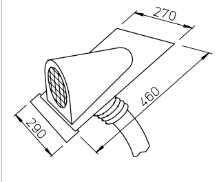
Maße SDH
