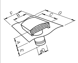
Maße DDF
