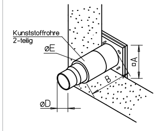
Maße TMK
