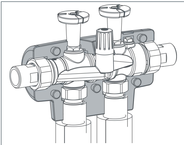
Abb. 4: Isolierschalen anbringen
