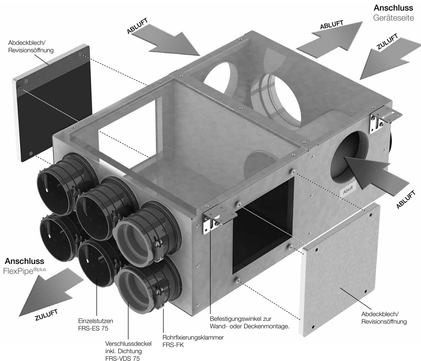
Abb.: Ausführung Zuluft links
