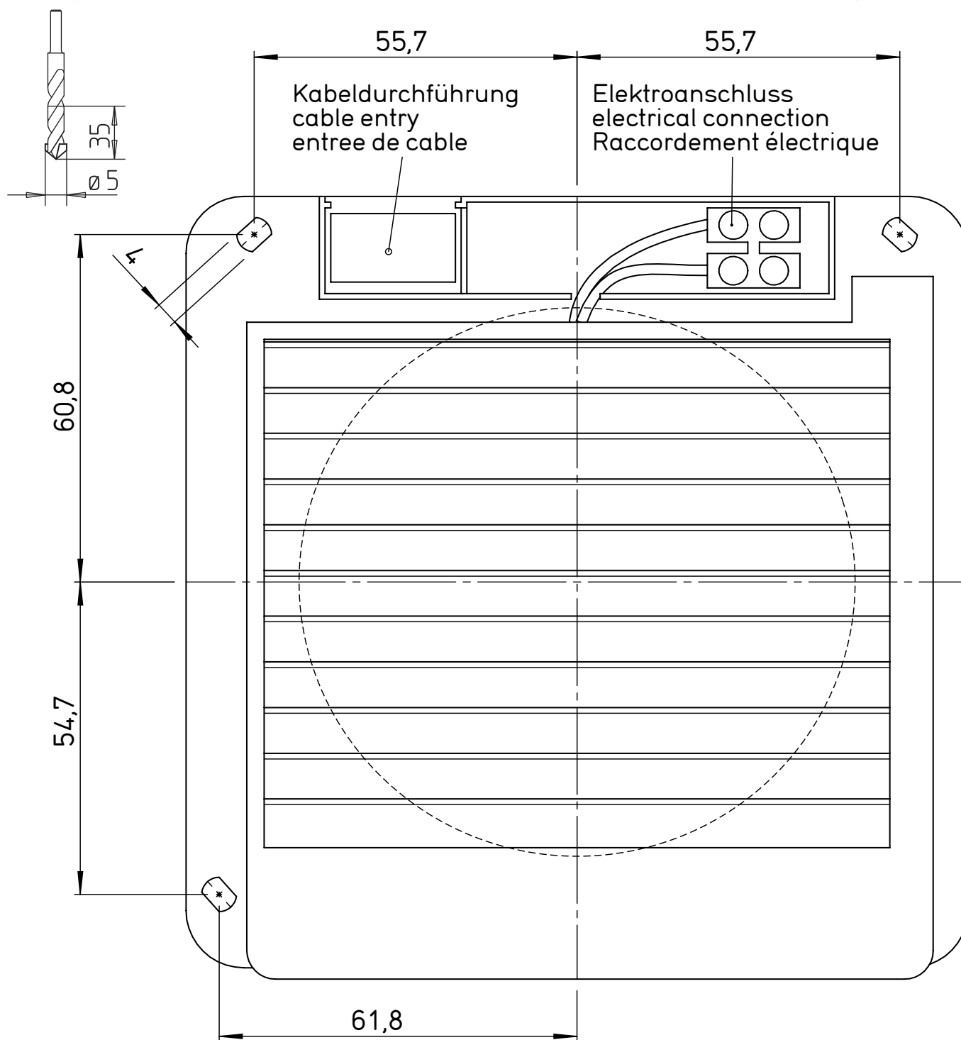
■ Montagebohrschablone EVK 100
