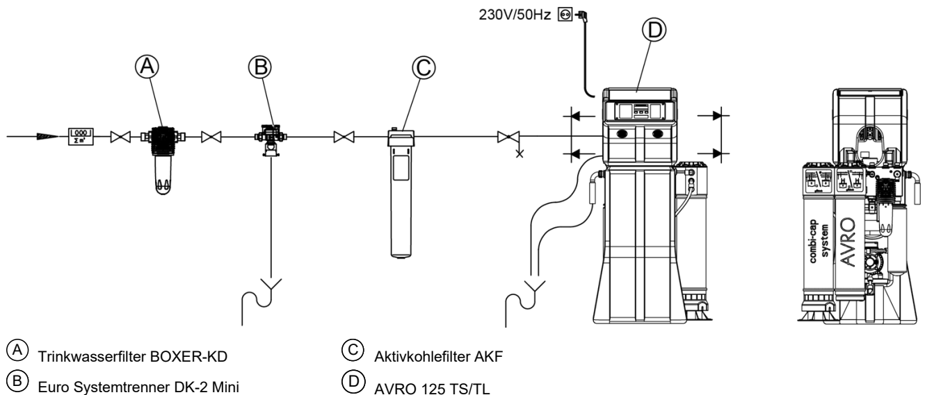
Abb. 2: Installationszeichnung
