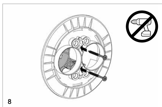
8. Verschrauben der Außenabdichtung [2] mit der Innenabdichtung [1].
