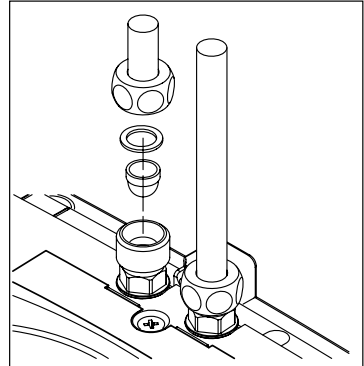
Fig. 11: «Skifte filtersil»
