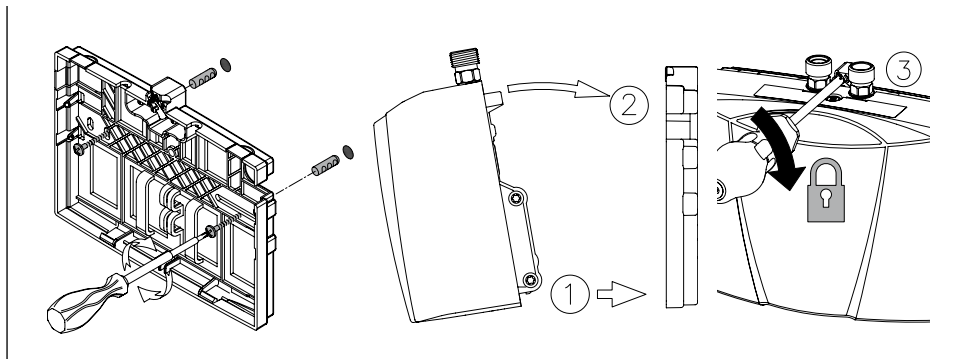
Kuva 5: "Seinäpidikkeen asennus"
