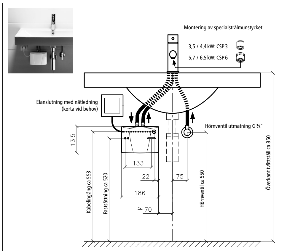
Bild 3: "Trykkløs (öppen) installation med armatur för trycklösa varmvattenberedare" (måttuppgifter i mm)
