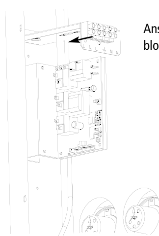
Mehrelement- Platine mit Anschlüssen (KA 40)
