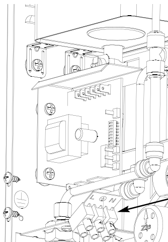
Einzelement- Platine mit Anschlüssen (KA 15/25)
