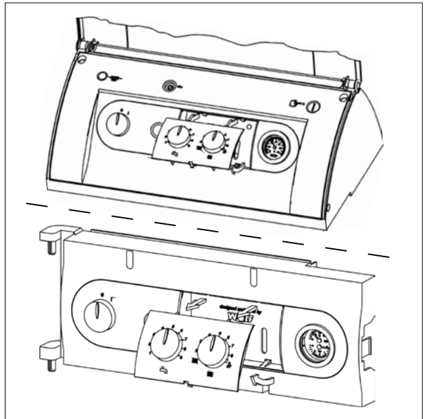
Abb. 4.8 Frontblende herausnehmen
