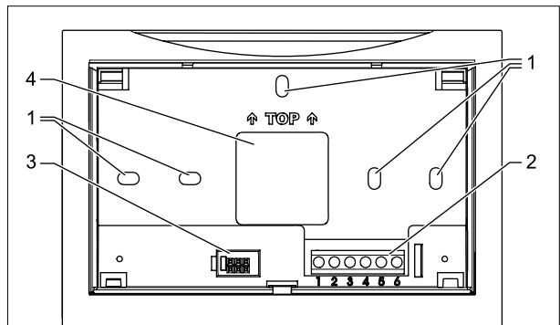
Abb. 4.5 Montage Wandschalter
