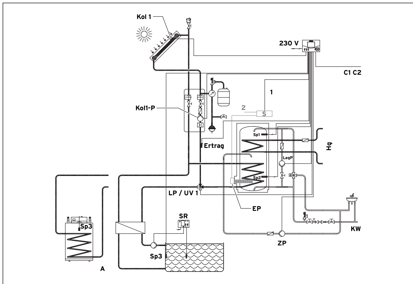
Abb. 5.3 Hydraulikplan 1: Anschluss zweiter Speicher oder Schwimmbad
