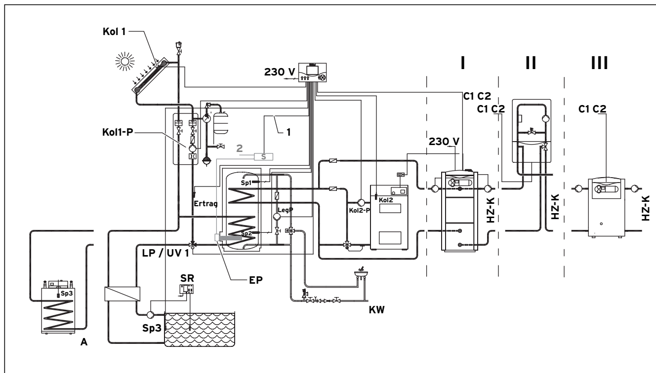
Abb. 5.13 Hydraulikplan 3: Anschluss zweiter Speicher oder Schwimmbad
