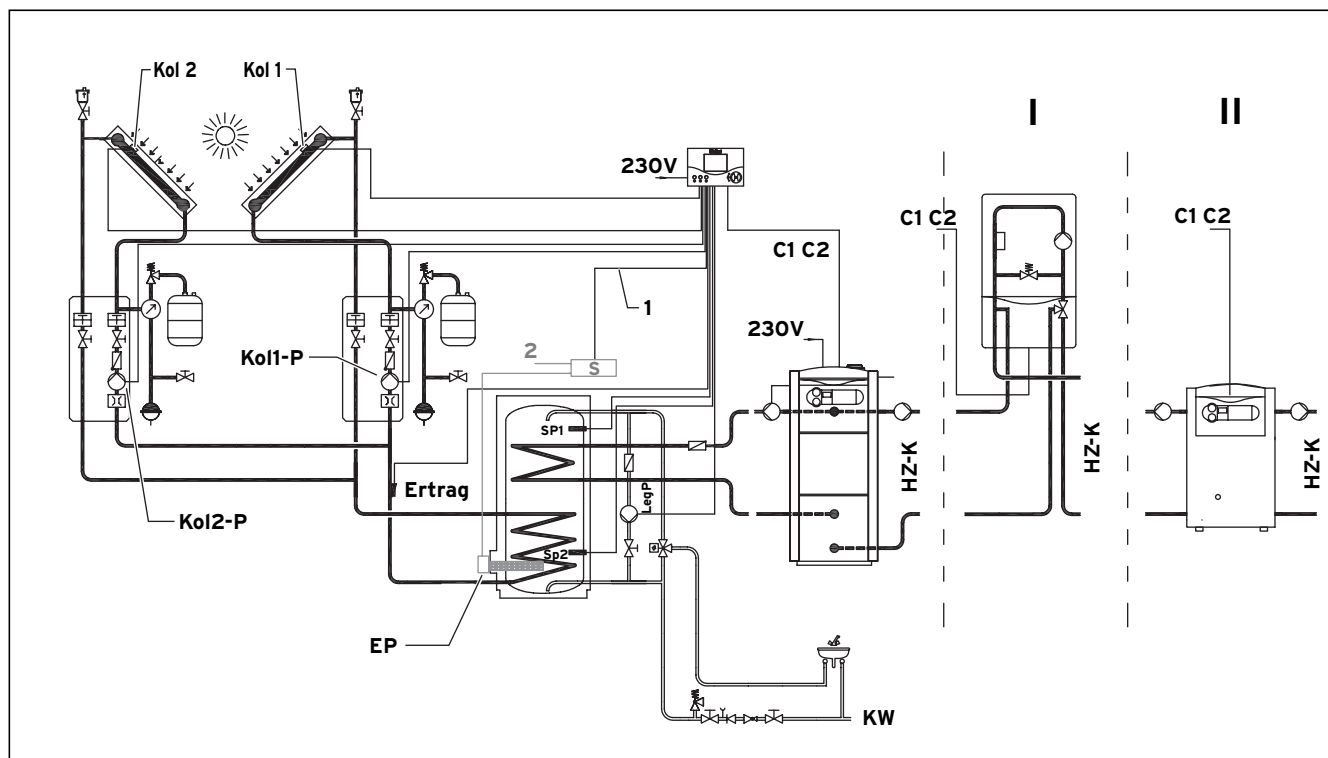
Abb. 5.7 Hydraulikplan 2 mit Anlagenkonfiguration: Zwei Kollektorfelder, ein Solarspeicher, Anschlussmöglichkeit von unterschiedlichen Wärmeerzeugern zum Nachladen des Speichers
