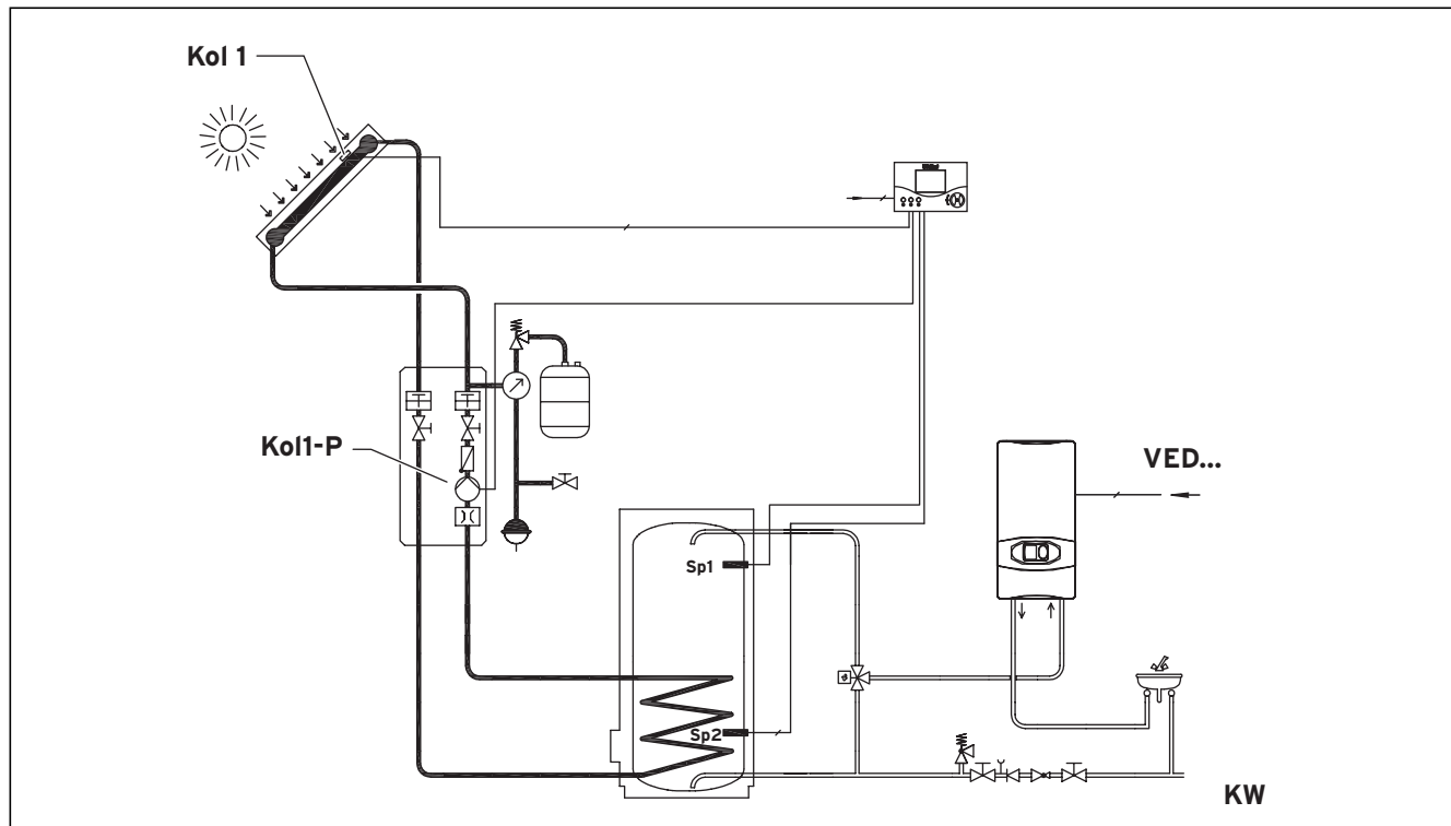
Abb. 5.5 Hydraulikplan 1: Einbindung in monovalente Systeme
