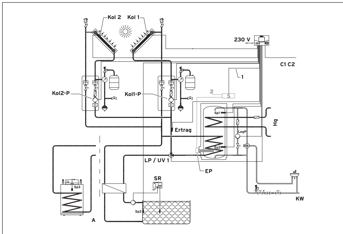
Abb. 5.9 Hydraulikplan 2: Anschluss zweiter Speicher oder Schwimmbad
