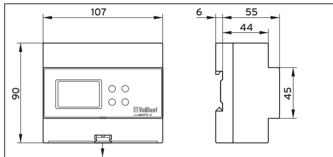
Abb. 4.1 Gehäuseabmessungen
