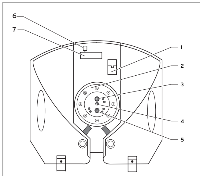
Abb. 10.1 Schaltraum
