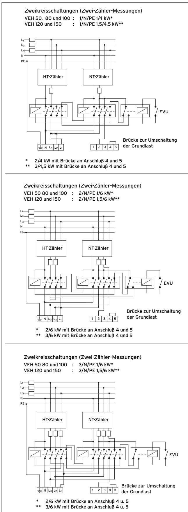
Abb. 8.3 Schaltschema (VEH exklusiv/pro)
