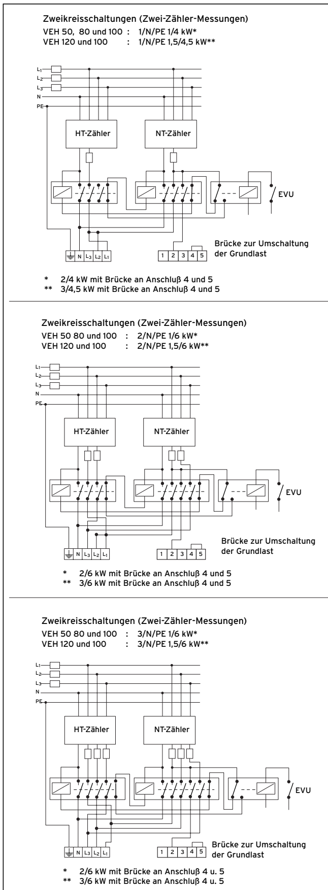
Abb. 8.3 Schaltschema (VEH exklusiv)
