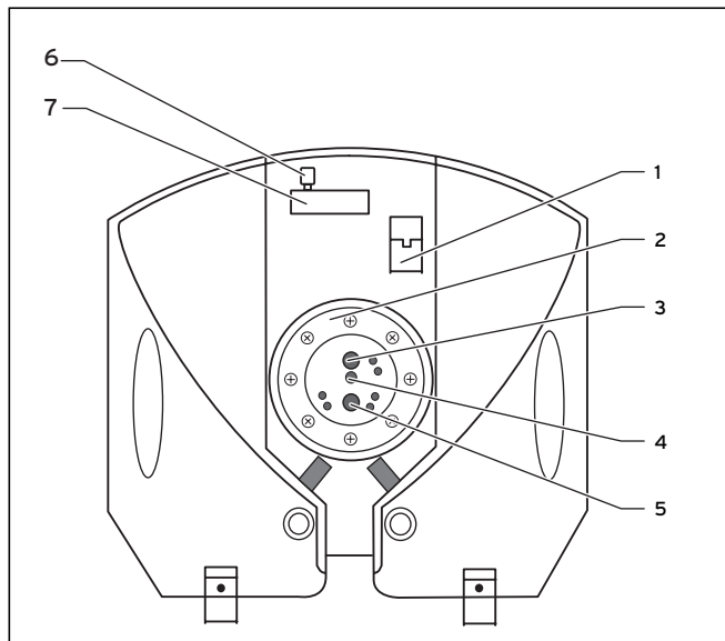
Abb. 10.1 Schaltraum
