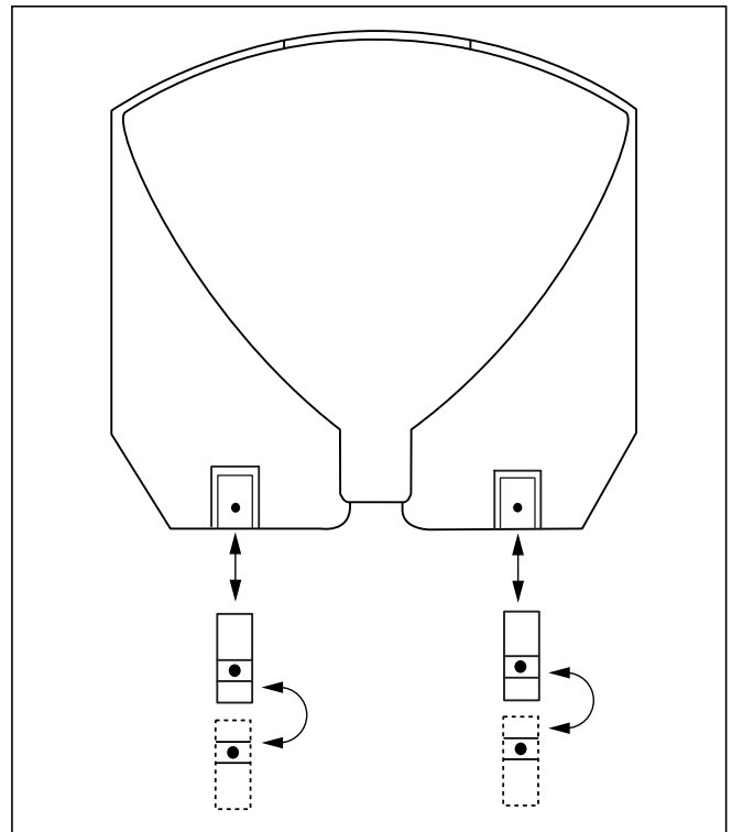
Abb. 7.2 Wandabsttzungen
