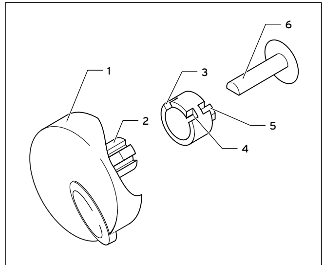
Abb. 9.1 Temperatureinstellbereich begrenzen
