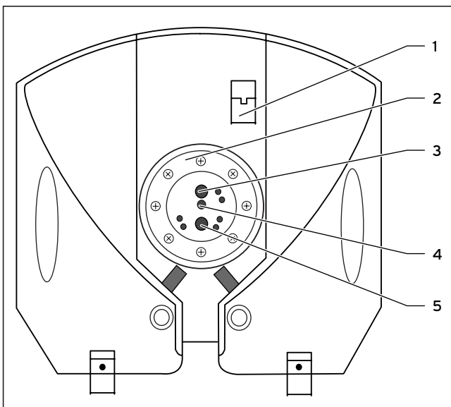
Abb. 7.1 Schaltraum
