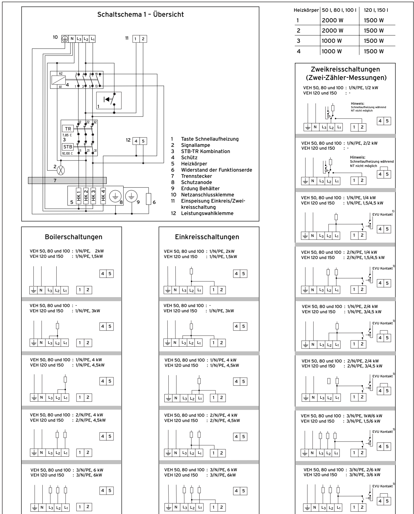
Abb. 5.2 Schaltschema (VEH exclusiv)
