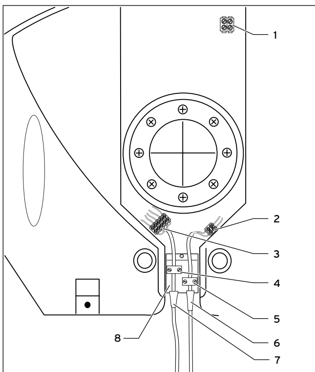
Abb. 5.1 Anschlusskasten
