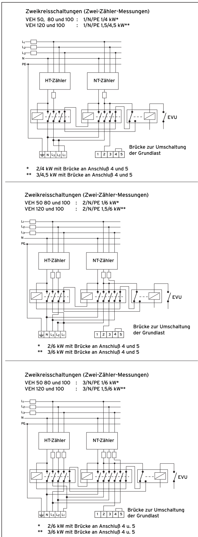
Abb. 5.3 Schaltschema (VEH exklusiv)
