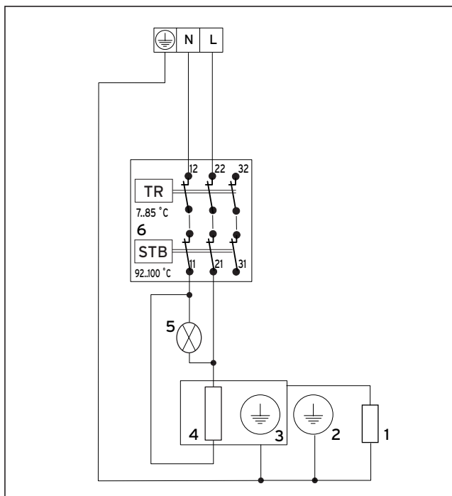
Abb. 5.2 Schaltschema (VEH classic)
