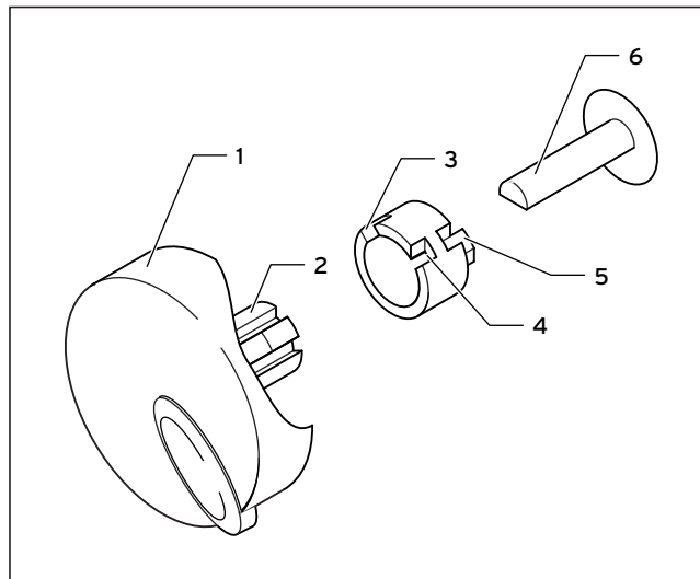
Abb. 6.1 Temperatureinstellbereich begrenzen
