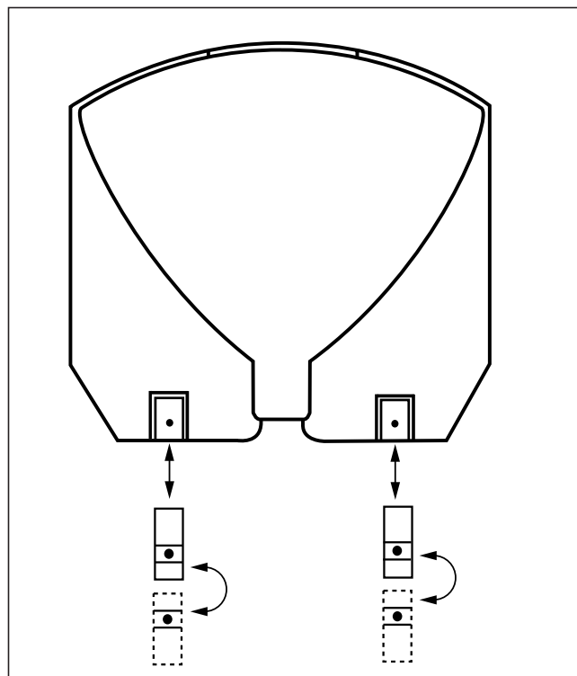
Abb. 4.1 Wandabstützungen
