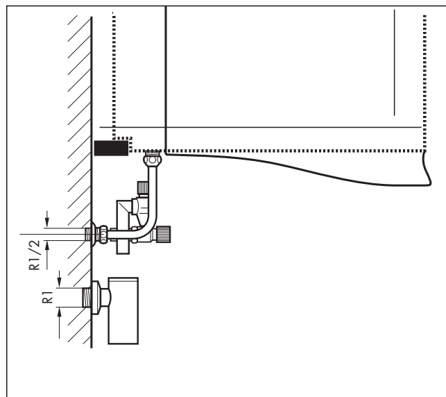
Abb. 4.4 Seitenansicht bei geschlossenem System
