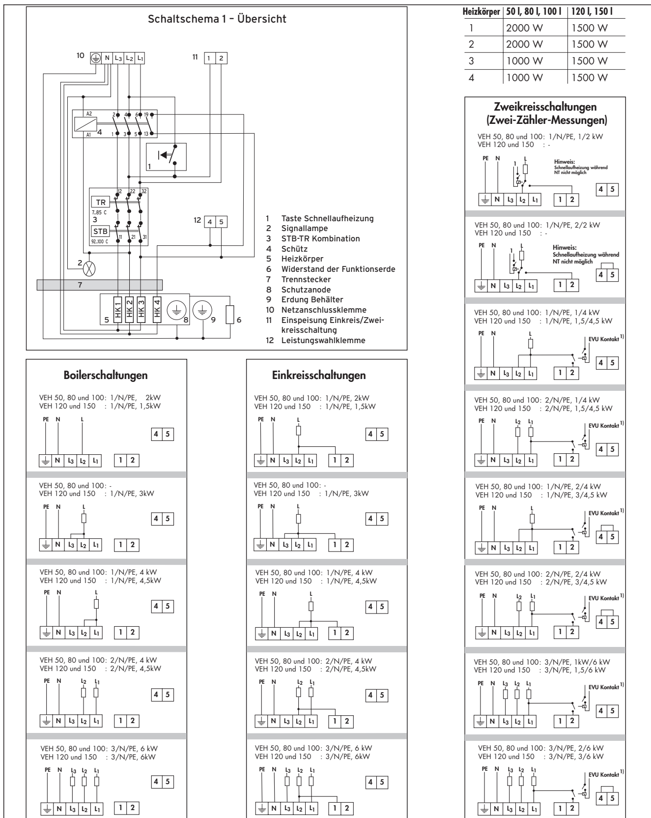
Abb. 5.2 Schaltschema (VEH exklusiv)
