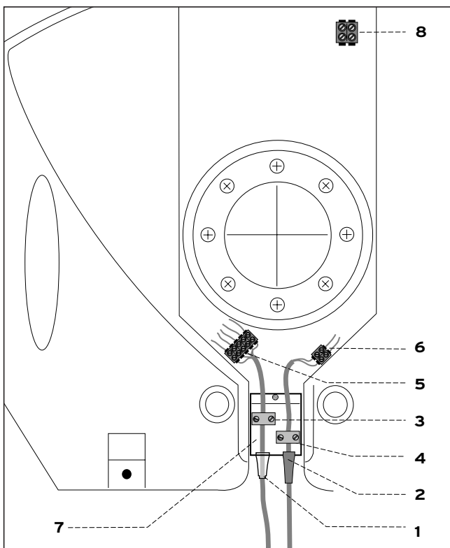
Abb. 5.1 Anschlußkasten
