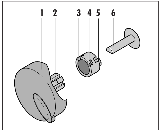
Abb. 6.1 Temperatureinstellbereich begrenzen
