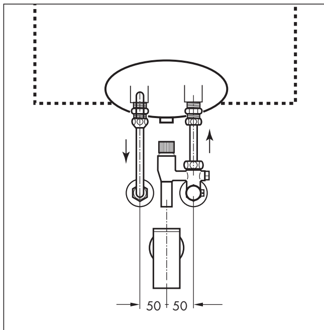
Abb. 4.3 Vorderansicht bei geschlossenem System (Maße in mm)
