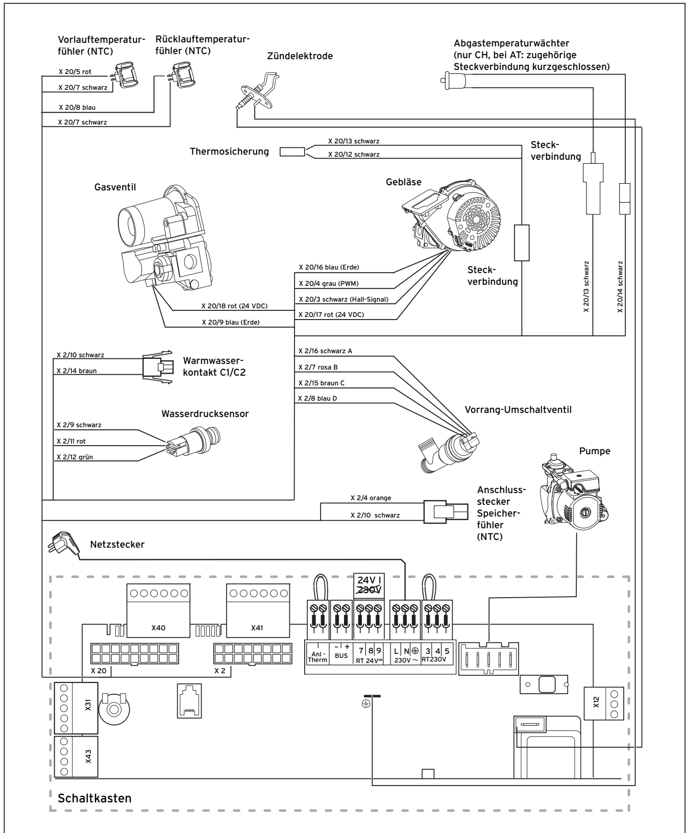
Abb. 4.2 Verdrahtung Brennwertgerät
