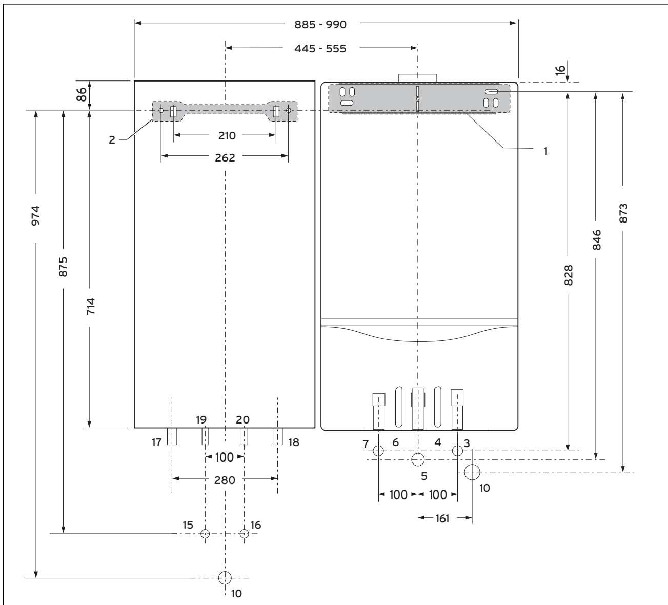
Мал. 3.2 Монтаж VІН СТ 70 поряд з конденсаційними опалювальними приладами
