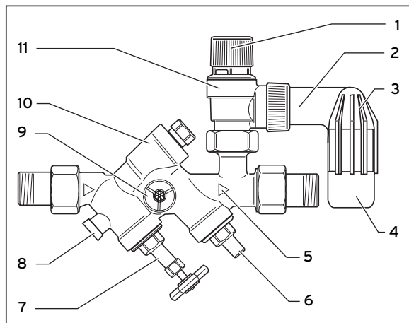
Рис. 1.1 Органы управления
