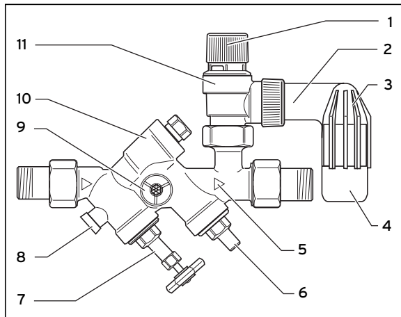
Fig. 1.1 Betjeningselementer
