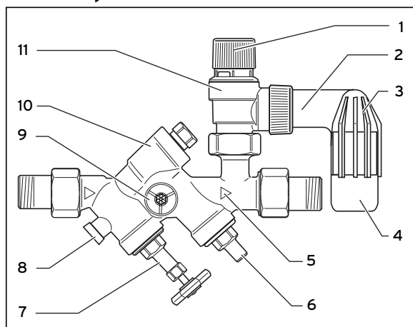
Rys. 1.1 Elementy obsługi
