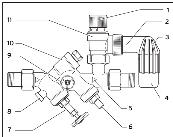
Abb. 1.1 Bedienungselemente
