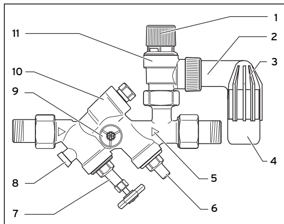
1.1. ábra Kezelőelemek
