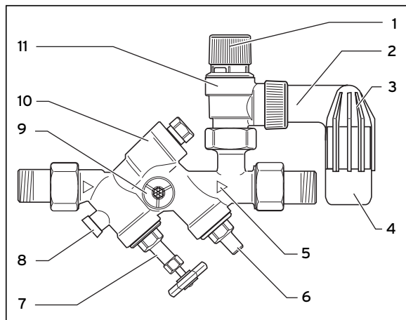
Obr. 1.1 Ovládací prvky
