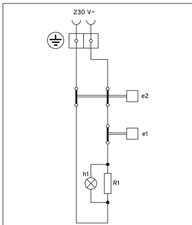
Abb. 7.1 Schaltplan
