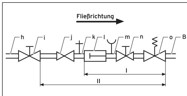
Abb. 6.3 Anschlussplan
