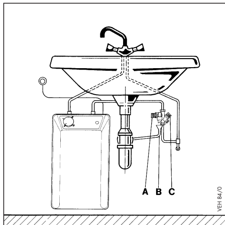
Abb. 1 Beispiel für geschlossene (druckfeste) Installation
