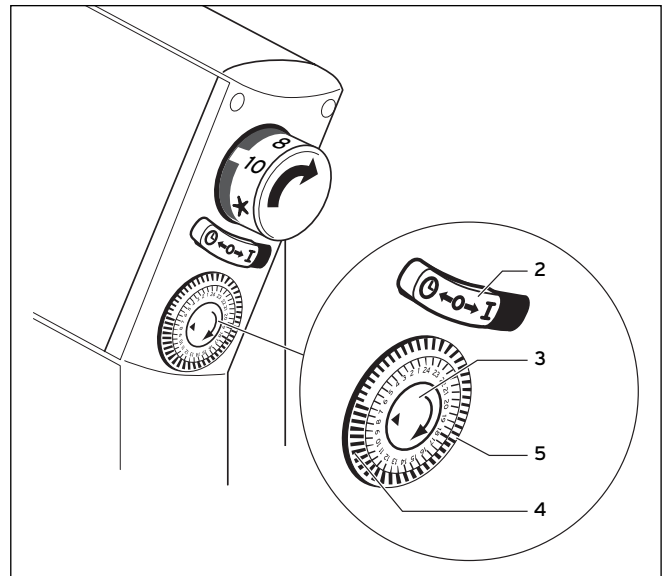
Abb. 6.3 24-Stunden-Zeitschaltuhr
