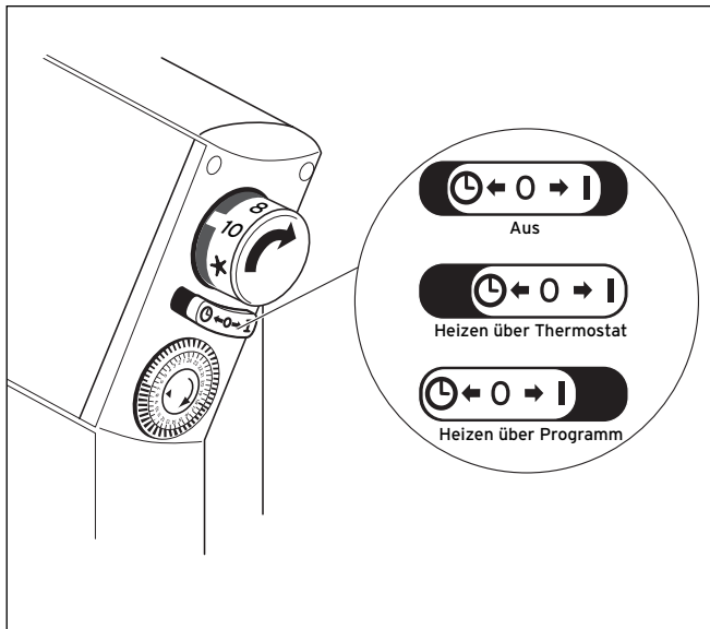
Abb. 6.2 Betriebsartenschalter
