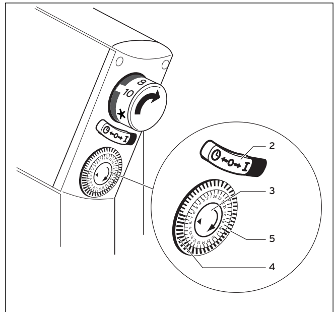
Abb. 6.3 24-Stunden-Zeitschaltuhr
