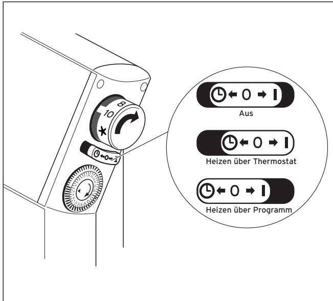
Abb. 6.2 Betriebsartenschalter
