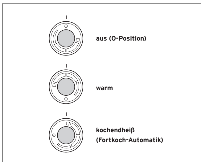
Abb. 3.2 Temperaturwähler
