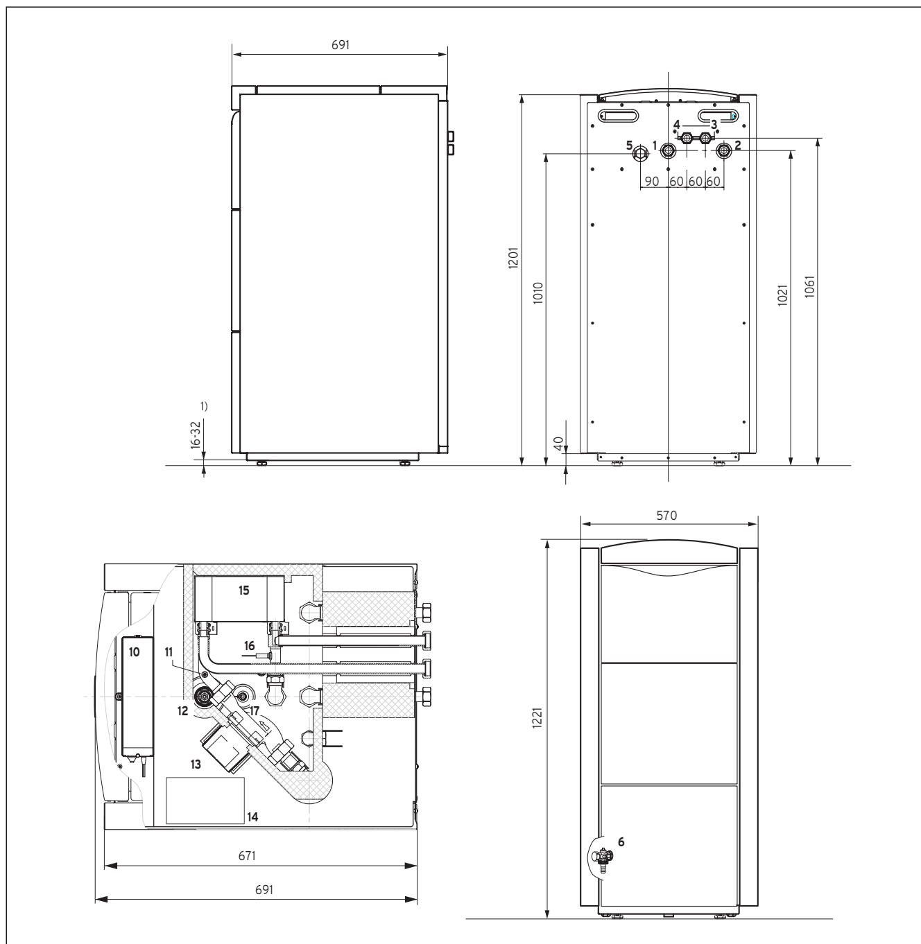
Abb. 5.2 Maßzeichnung
