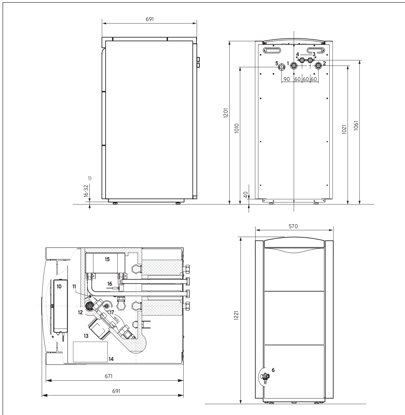
Afb. 5.2 Maattekening
