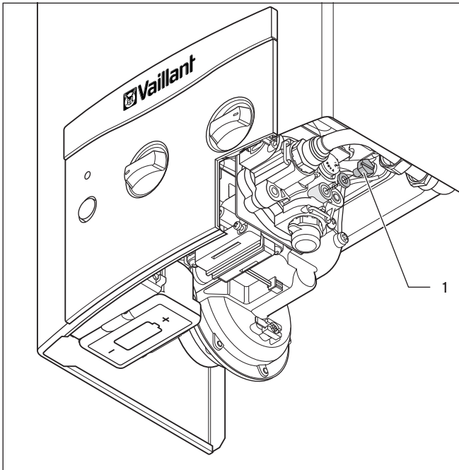
Abb. 4.7 Entleerung
