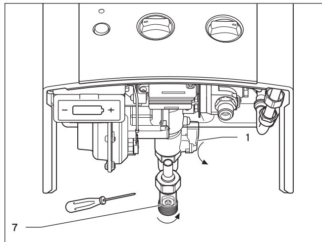
Abb. 4.2 Absperrvorrichtungen
