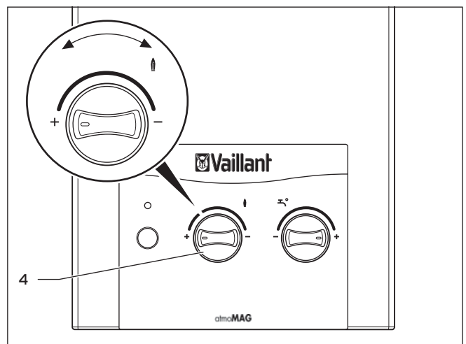
Abb. 4.5 Leistungsvorwahl
