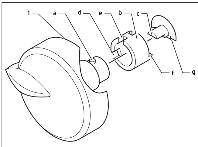
Abb. 7.1 Temperaturwähler
