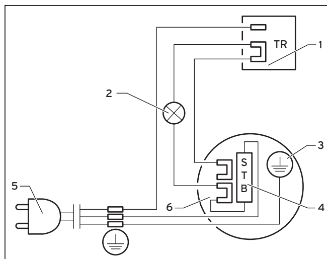
Fig. 4.8 Schéma électrique
