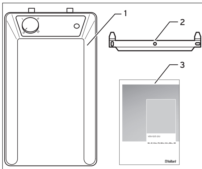
Abb. 4.1 Lieferumfang VEN 10/5 U Untertischgerät
