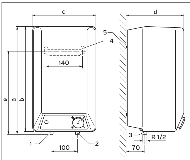
Abb. 4.6 Abmessungen VEN 10/5 0
